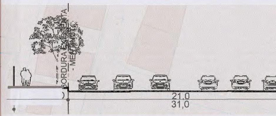
A-A SOS. VERGULUI - PROFIL PROPOS
