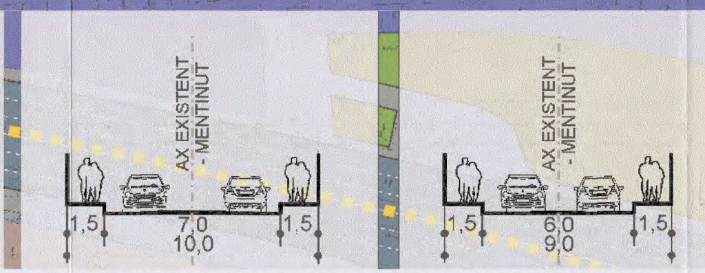
E-E STRAZI DE DESERVIRE LOCALA - PROFIL EXISTENT - MENTINUT
