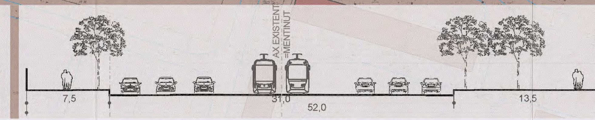
B-B SOS. PANTELIMON - PROFIL EXISTENT - MENTINUT
