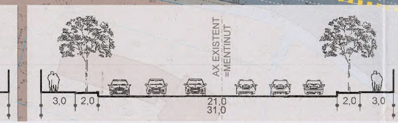
C-C DUL BASARABIA - PROFIL EXISTENT - MENTINUT
