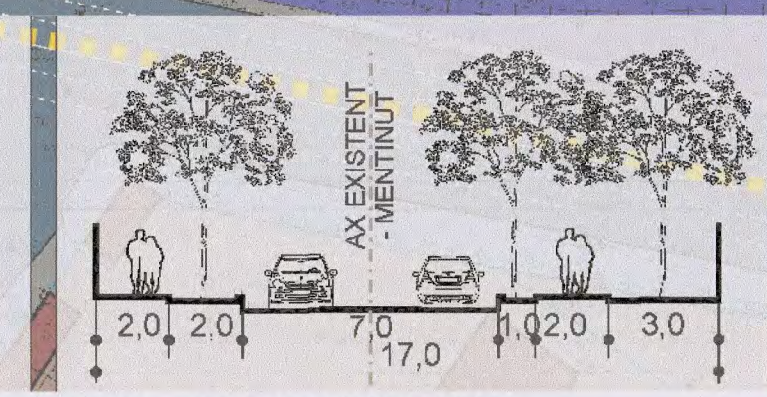
D-D STR. ION SAHIGHIAN - PROFIL EXISTENT - MENTINUT
