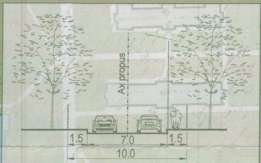
Profil A-A (Strada propusa) sc. 1:200
