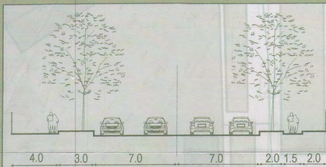
Profil Str. Emil Racovita existent si mentinut - sc. 1:200
