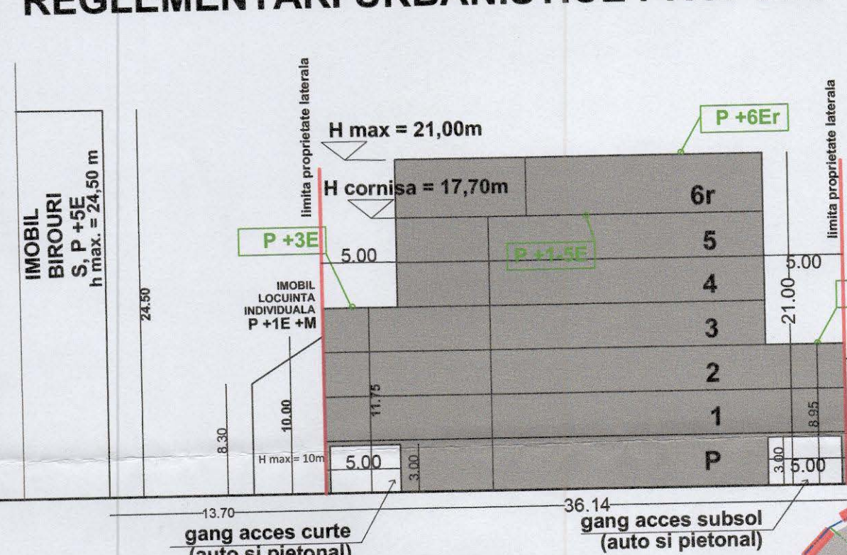
SECTIUNE A - A', SITUATIE PROPUZA PROFIL LONGITUDINAL STR. TABACARILOR
