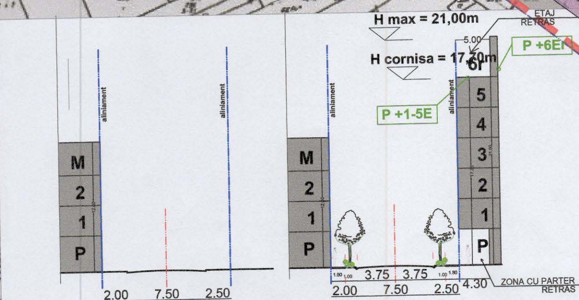
SECTIUNE C - C', SITUATIE PROPUZA - PROFIL TRANSVERSAL STR. TABACARILOR
