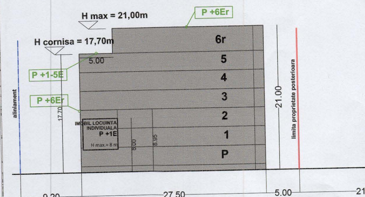
SECTIUNE B - B', SITUATIE PROPUZA - PROFIL TRANSVERSAL STR. TABACARILOR
