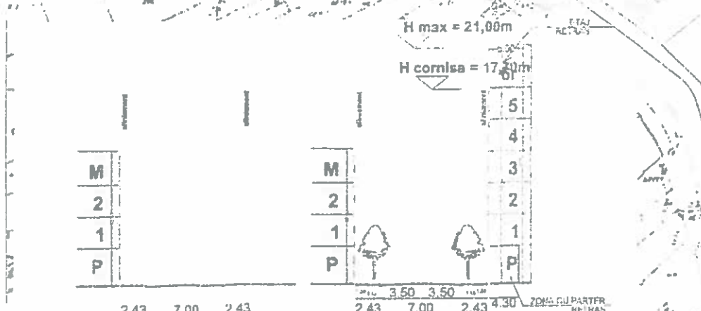
SITUATIE EXISTENTA - PROFIL TRANSVERSAL STR. TABACARILOR
