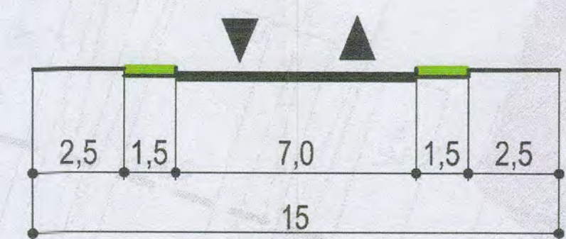
Profil transversal 1-1
