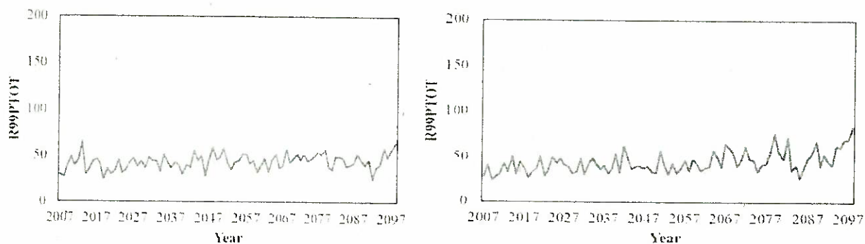
Fig. 2.2.1-10 Evoluția sumei anuale a precipitațiilor căzute în zilele în care precipitația maximă zilnică depășește percentila de 99 a cantității zilnice de precipitații din perioada 2007-2098 în condițiile scenariilor RCP 4.5 (stânga) și RCP 8.5 (dreapta) pentru Municipiul București.
