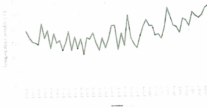
Figura 2.2.1-7 Evoluția temperaturii medii anuale (°C) la stațiile meteorologice București-Băneasa și București-Filaret, 1961-2020
