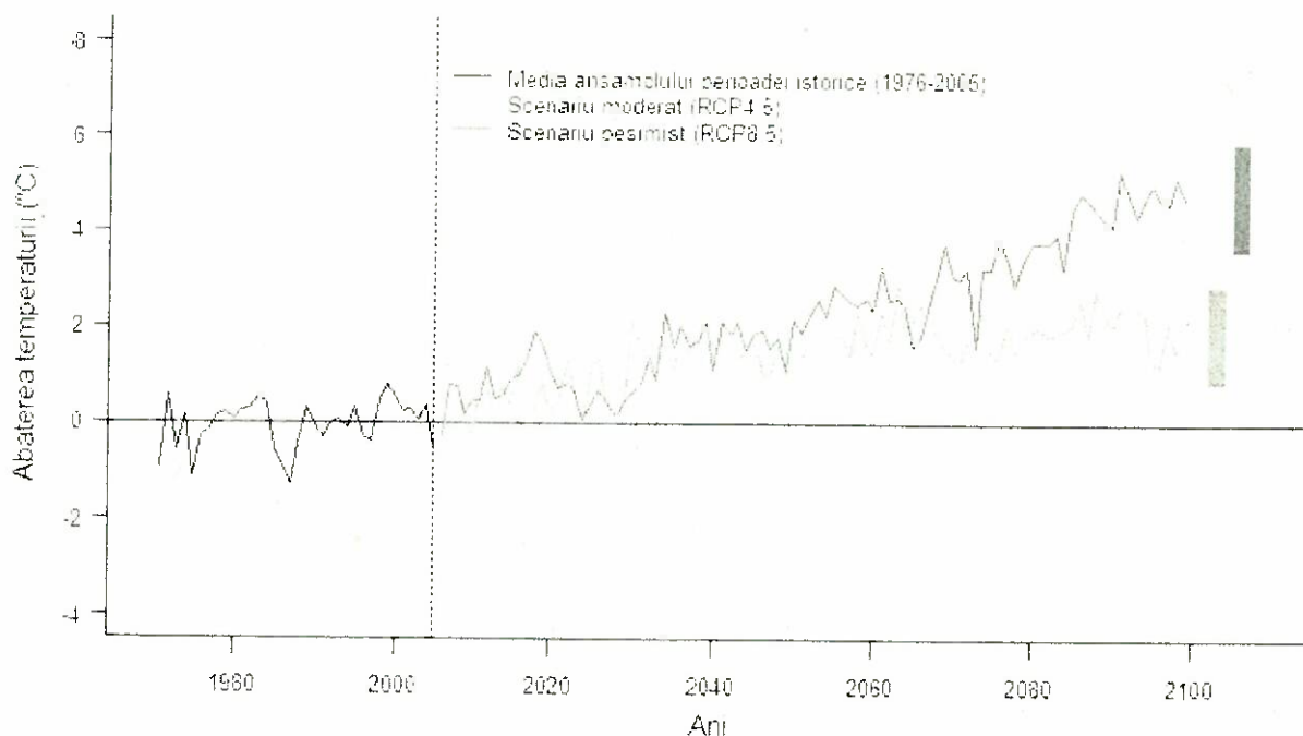
Fig. 2.2.1-9 Abaterea temperaturii aerului pentru diferite orizonturi de timp, față de media perioadei istorice, în Municipiul București, în condițiile scenariilor climatice RCP 4.5 și RCP 8.5.
