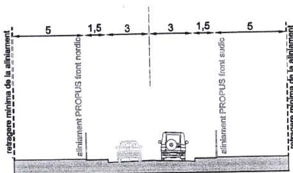
PROFIL 2-2
