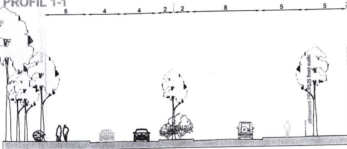
PROFIL 1-1
