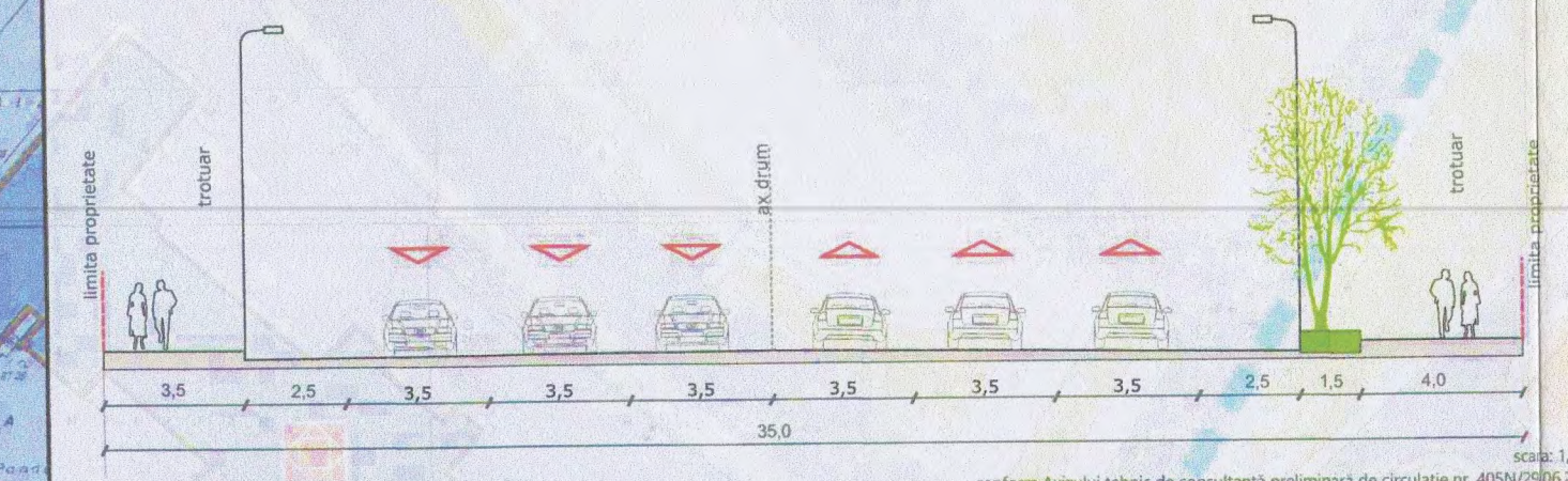
B-B Strada Progresului (profil existent)
