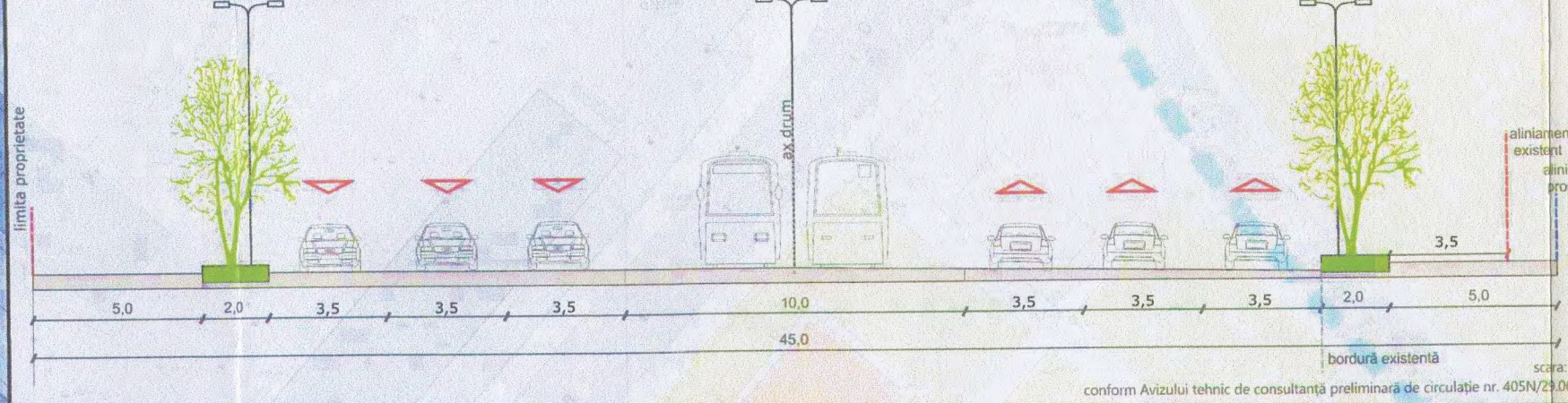
B'-B Strada Progresului (profil propus - PUZ Spătaru Preda nr. 2 conform Avizului tehnic de consultanță preliminară de circulație nr. 405N/29.06.2018)
