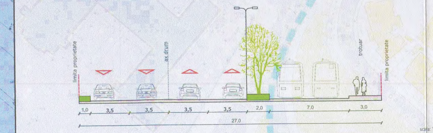
B'-B Strada Progresului (profil propus - PUZ Spătaru Preda nr. 2 conform Avizului tehnic de consultanță preliminară de circulație nr. 405N/29.06.2018)
