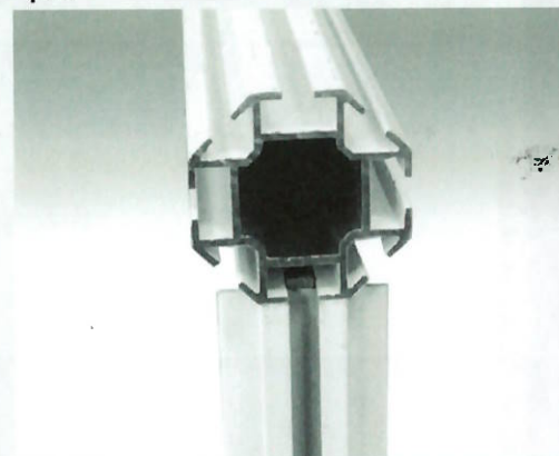
Model conexiune bara paze - montant
