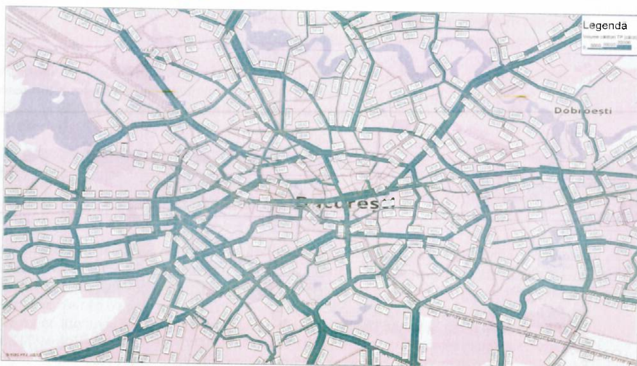
Figura 4.5-2. Alocarea fluxurilor de călători pe rețeaua de transport public de suprafață – Anul 2025 (sursa: Modelul de transport)
