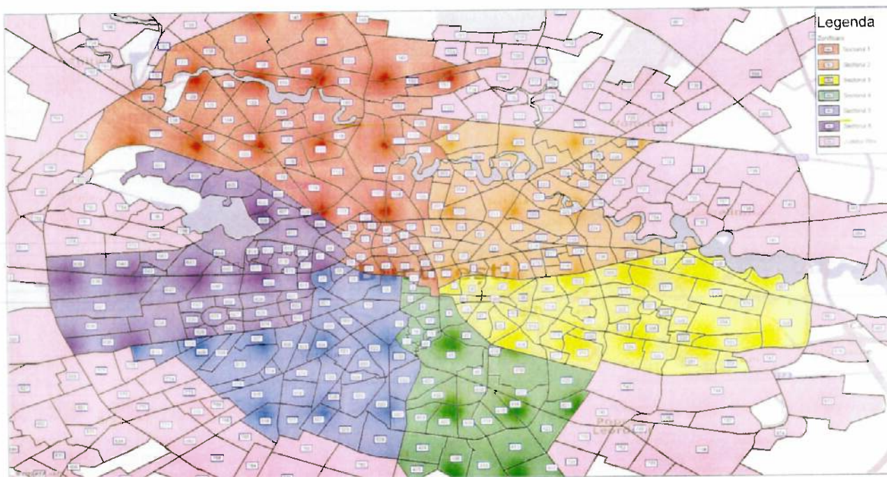
Figura 4.2-3. Sistemul de zonificare a modelului de transport (sursa: Modelul de transport)
