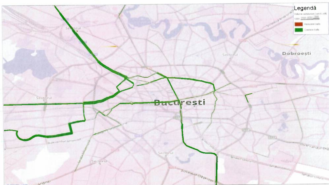
Figura 6.2-7. Diferențe Volume de trafic, Transport public, Scenariul cu Proiect, 2029 (Sursa: Modelul de transport)
