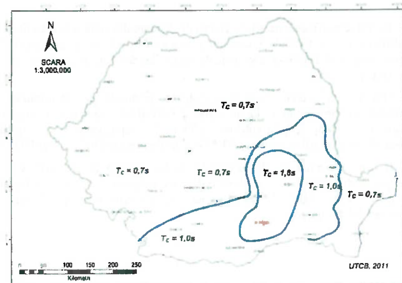
Figura 3 - Zonarea teritoriului României în termeni de perioadă de control (colț) T_c a spectrului de răspuns
