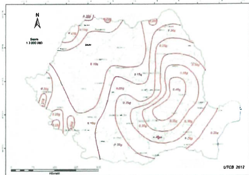
Figura 2 - Zonarea valorilor de vârf de accelerație terenului pentru proiectare a_g=0.225g și 20% probabilitate de depășire în 50 de ani
