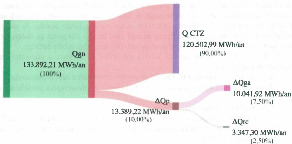
Figura 16.2 – Diagrama Sankey – bilanțul termooenergetic optimizat al CTZ Titan
