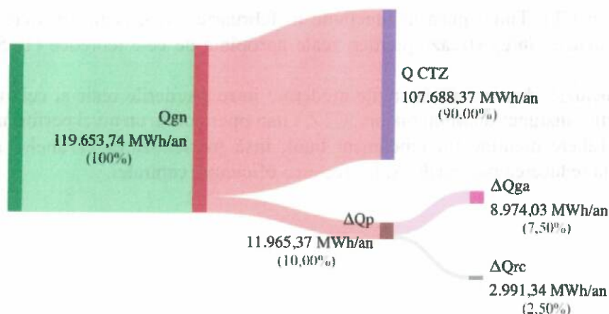
Figura 14.1 – Diagrama Sankey – bilanțul termooenergetic tehnologic pentru CTZ CPL, anul 2024
