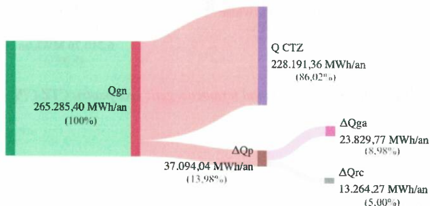
Figura 12.3 – Diagrama Sankey – bilanțul termoeenergetic real pentru CTZ CPL și CTZ Titan, anul 2024
