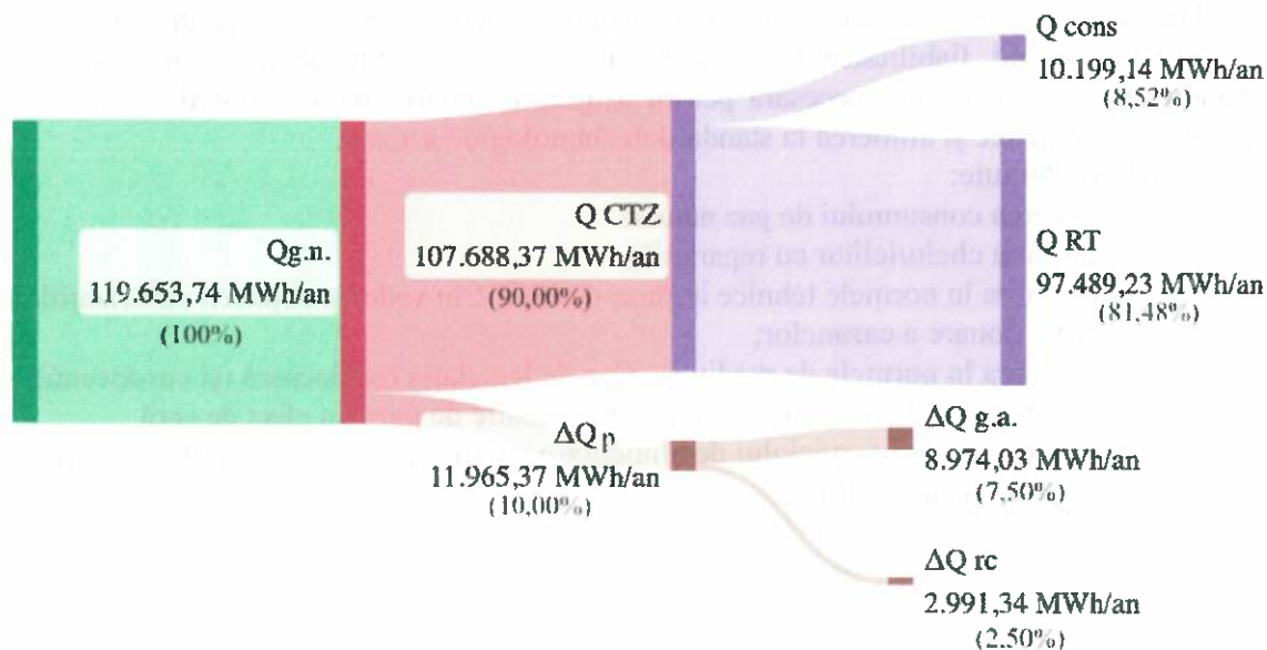
Figura 16.1 – Diagrama Sankey – bilanțul termooenergetic optimizat al CTZ CPL
