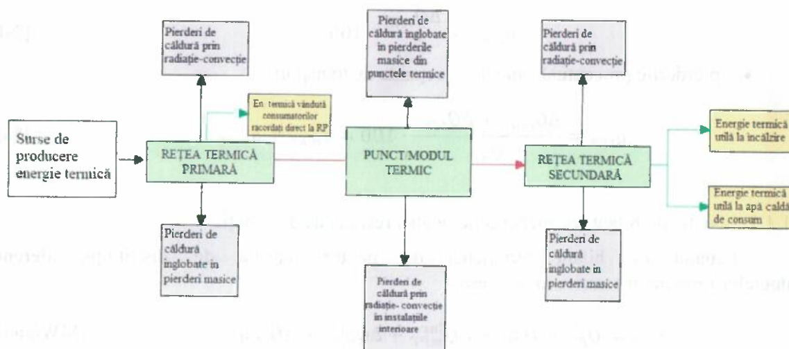
Figura 11.1 – Schema fluxurilor energetice din conturul rețelei de transport și distribuție aferentă punctelor și modulelor termice
