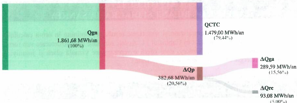
Figura 12.2 – Diagrama Sankey – bilanțul termooenergetic anual real pentru CTC fără RD, anul 2024
