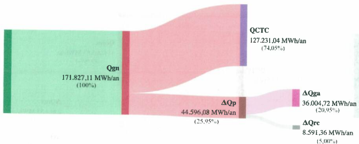
Figura 12.1 – Diagrama Sankey – bilanț termooenergetic anual real pentru CTC cu RD, anul 2024
