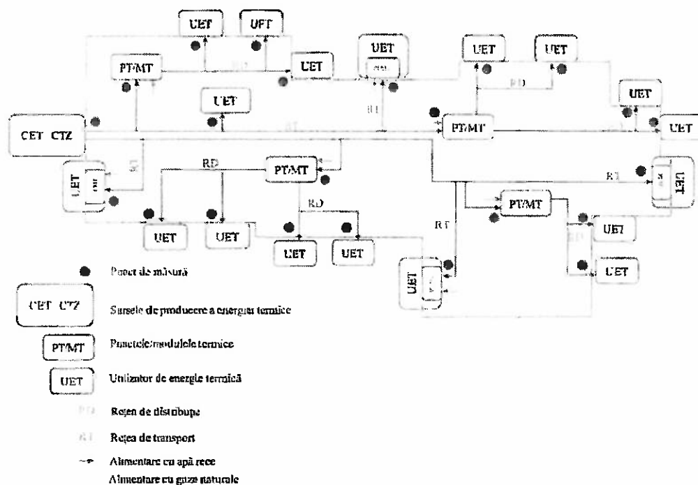
Figura 2 – Schema fluxului tehnologic din conturul de bilanț al rețelelor de transport și distribuție aferente PT/MT și punctele de măsură identificate
