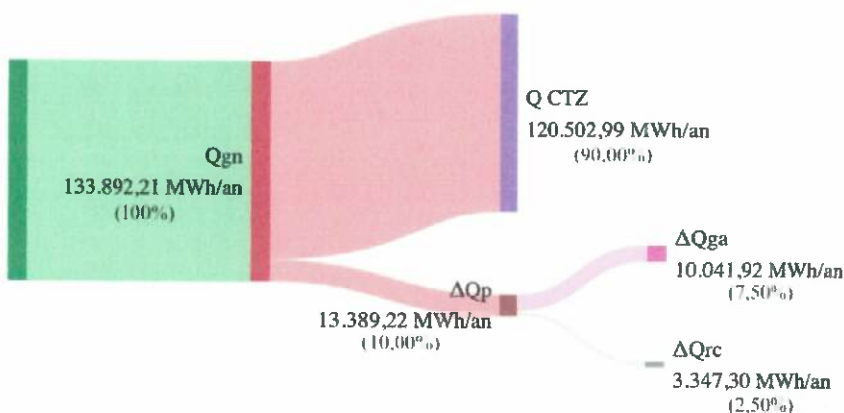
Figura 14.2 – Diagrama Sankey – bilanțul termooenergetic tehnologic pentru CTZ Titan, anul 2024
