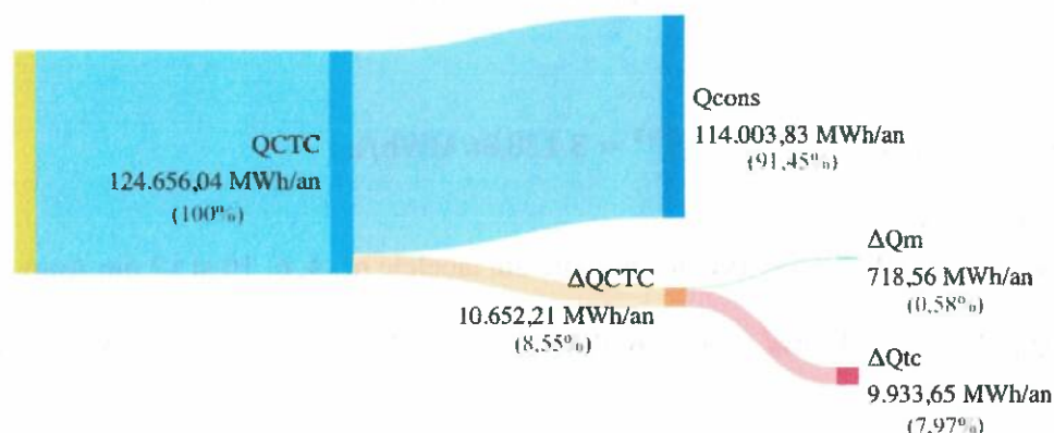
Figura 14.3 – Diagrama Sankey – bilanțul termooenergetic tehnologic pentru RD aferentă CTC, anul 2024
