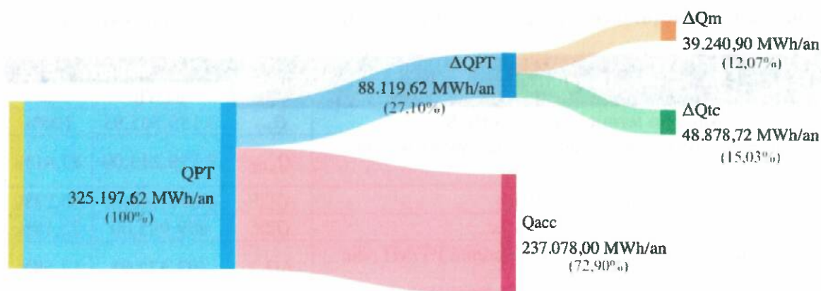
Figura 12.5 – Diagrama Sankey – bilanțul termoeenergetic real pentru RD aferentă PT/MT, sezonul cald, anul 2024
