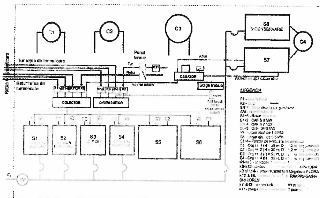
Figura 1 – Schema de funcționare a CTZ CPL
