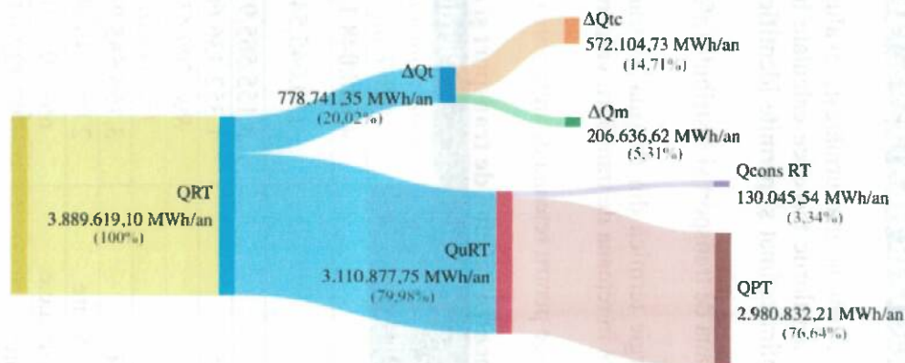
Figura 14.1 – Diagrama Sankey – bilanțul termoeenergetic tehnologic pentru RT, anul 2024
