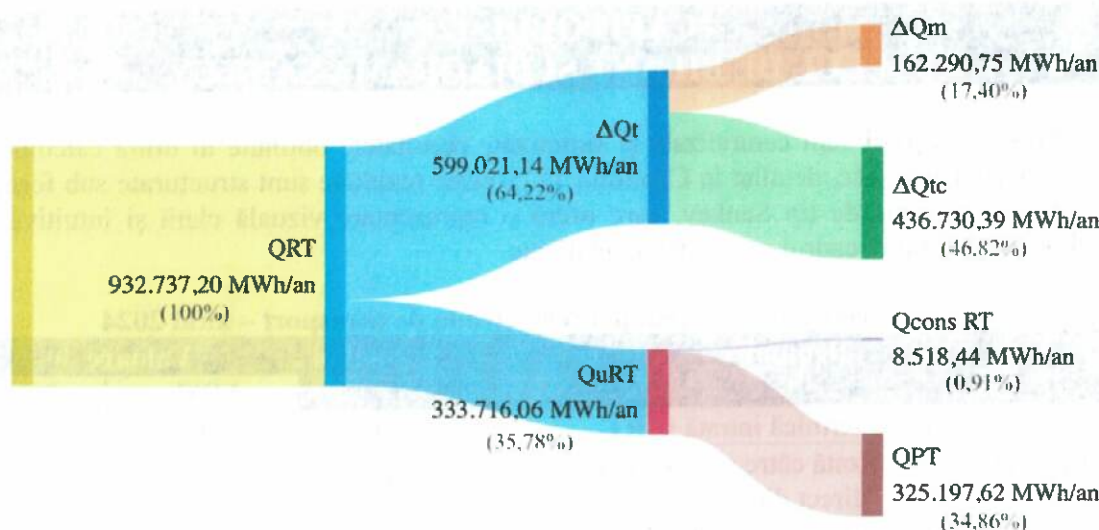
Figura 12.2 – Diagrama Sankey – bilanțul termoeenergetic real pentru RT, sezonul cald, anul 2024
