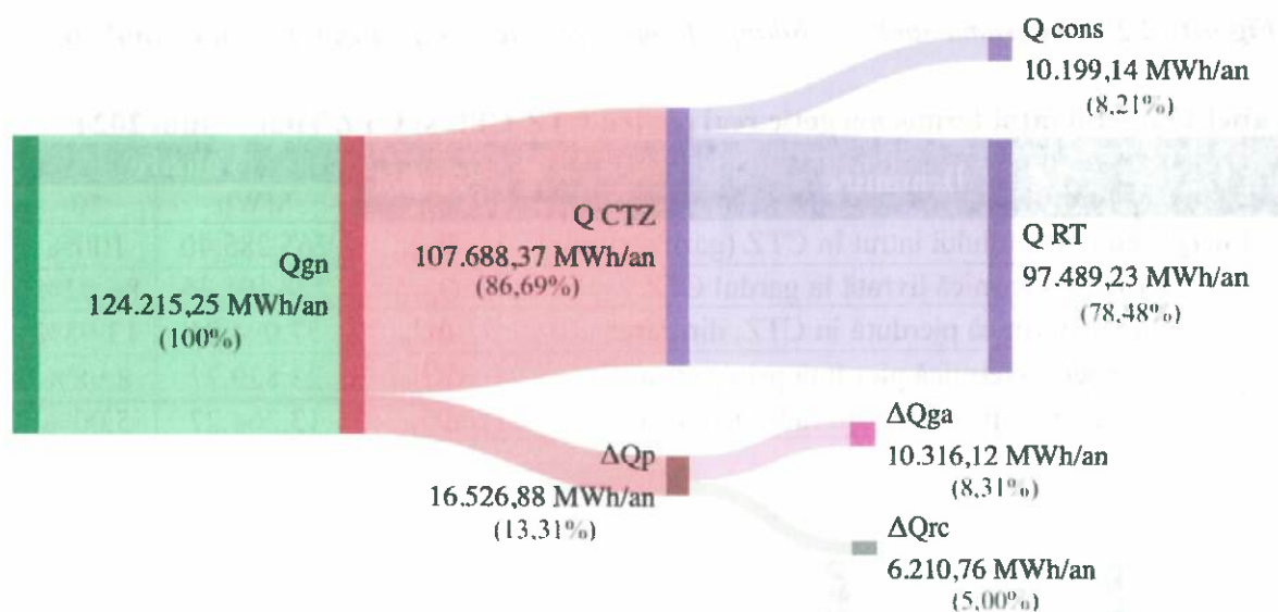
Figura 12.1 – Diagrama Sankey – bilanțul termoeenergetic real pentru CTZ CPL, anul 2024
