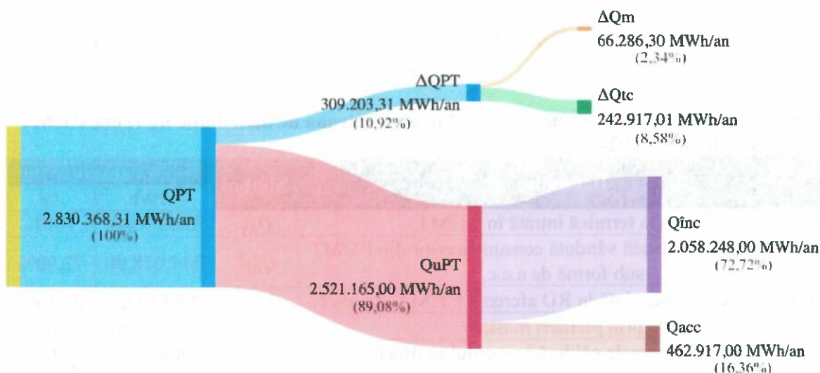
Figura 12.6 – Diagrama Sankey - bilanțul termoeenergetic real pentru RD aferentă PT/MT, sezonul cald, anul 2024
