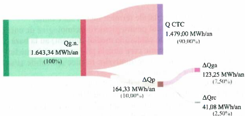
Figura 14.2 – Diagrama Sankey – bilanțul termooenergetic tehnologic pentru CTC fără RD, anul 2024
