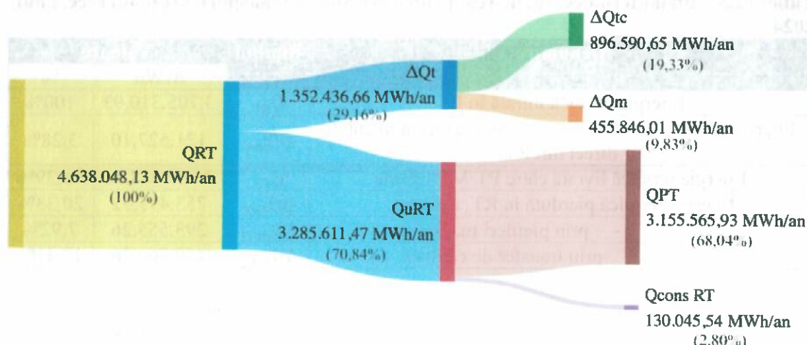
Figura 12.1 – Diagrama Sankey – bilanțul termooenergetic real pentru RT, anul 2024
