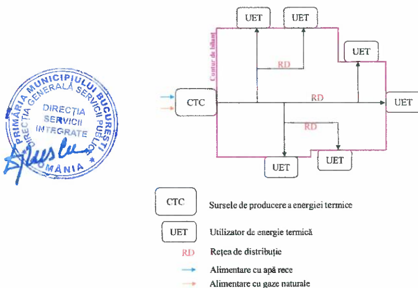
Figura 5.2 – Schema fluxului tehnologic din conturul de bilanț al CTC cu RD aferente
