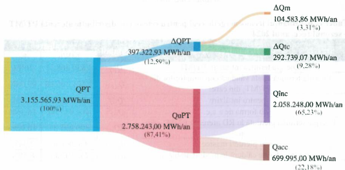
Figura 12.4 – Diagrama Sankey – bilanțul termoeenergetic real pentru RD aferentă PT/MT, anul 2024
