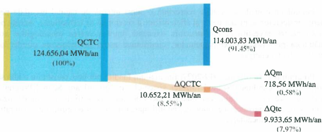
Figura 17.1 – Diagrama Sankey – bilanțul termooenergetic optimizat pentru RD aferentă CTC
