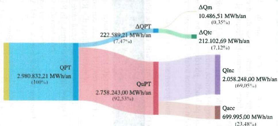
Figura 14.2 – Diagrama Sankey – bilanțul termoeenergetic tehnologic pentru RD aferentă PT/MT, anul 2024
