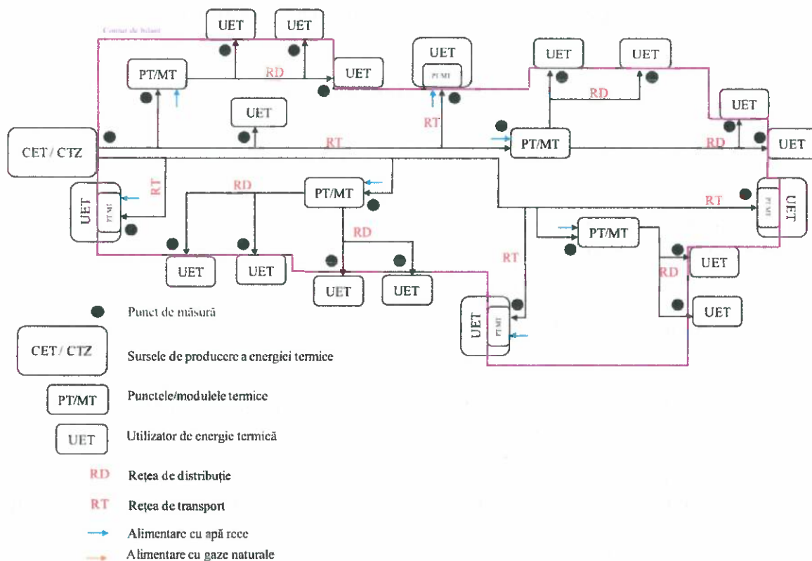
Figura 9.1 – Schema fluxului tehnologic din conturul de bilanț al RT și RD și punctele de măsură identificate
