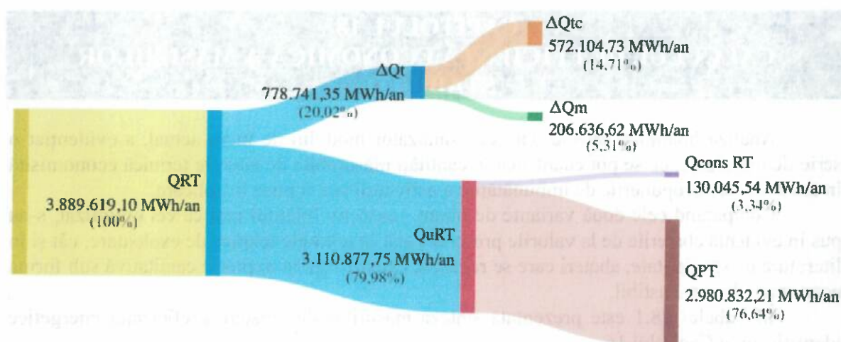
Figura 17.1 – Diagrama Sankey pentru regimul optimizat de funcționare a rețelei de transport
