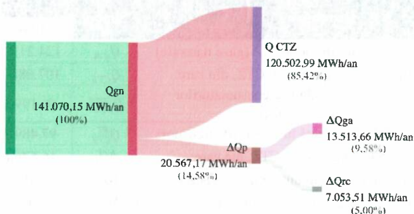
Figura 12.2 – Diagrama Sankey – bilanțul termoeenergetic real pentru CTZ Titan, anul 2024
