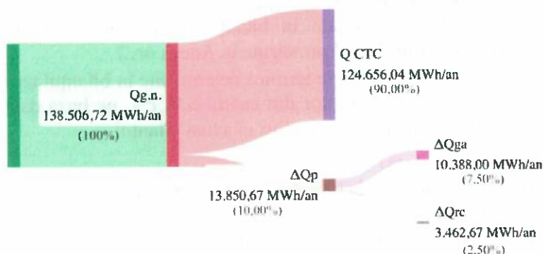
Figura 14.1 – Diagrama Sankey – bilanțul termooenergetic tehnologic pentru CTC cu RD, anul 2024
