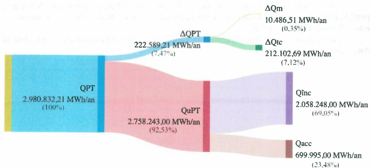
Figura 17.2 – Diagrama Sankey pentru regimul optimizat de funcționare a rețelei de distribuție aferentă PT/MT
