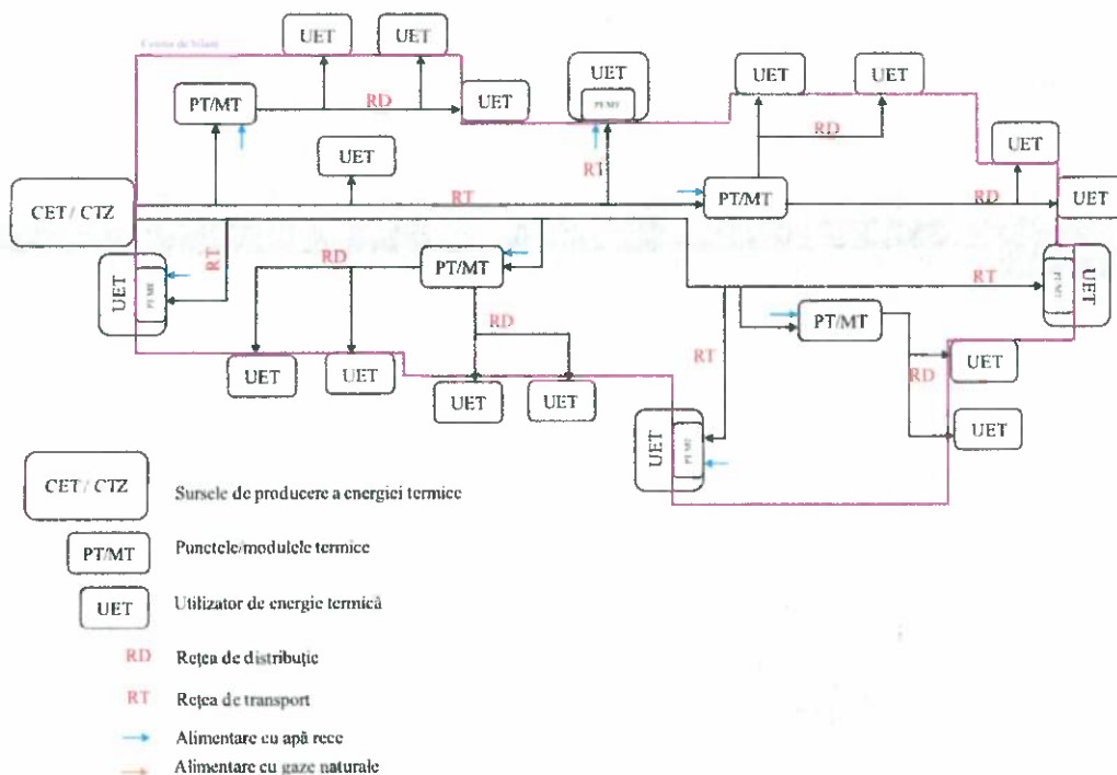
Figura 5.1 – Schema fluxului tehnologic din conturul de bilanț al RT și RD
