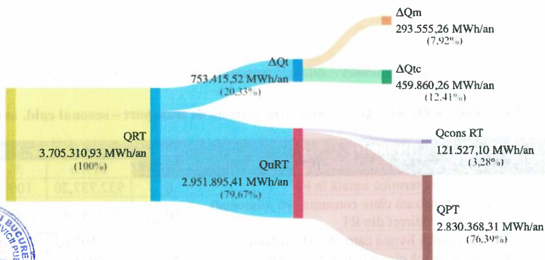
Figura 12.3 – Diagrama Sankey – bilanțul termoeenergetic real pentru RT, sezonul rece, anul 2024
