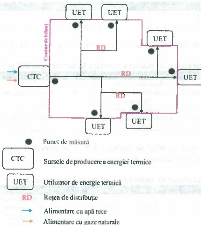
Figura 9.2 – Schema fluxului tehnologic din conturul de bilanț al CTC cu RD aferente și punctele de măsură identificate
