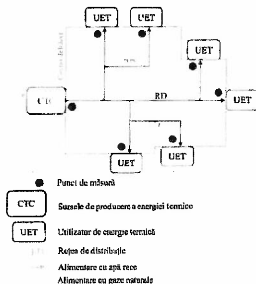
Figura 3 – Schema fluxului tehnologic din conturul de bilanț al CTC cu rețelele de distribuție aferente și punctele de măsură identificate
