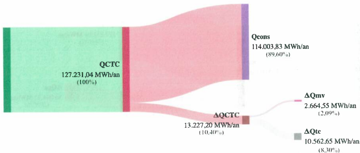
Figura 12.3 – Diagrama Sankey – bilanțul termooenergetic anual real pentru RD aferentă CTC, anul 2024
