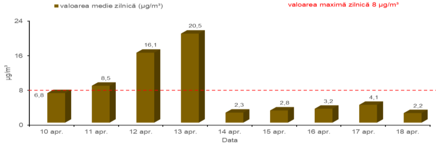
Valorile medii zilnice ale concentrațiilor de hidrogen sulfurat (H 2 S) Perioada: 10.04 - 18.04.2021 Depou STB Giurgiului, sector 4
