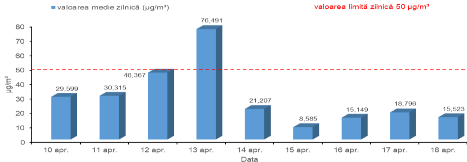
Valorile medii zilnice ale concentrațiilor de particule în suspensie PM10 Perioada: 10.04 - 18.04.2021 Depou STB Giurgiului, sector 4
