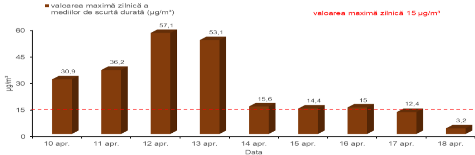
Valorile maxime zilnice a mediilor de scurtă durată ale concentrațiilor de hidrogen sulfurat (H 2 S) Perioada: 10.04 - 18.04.2021 Depou STB Giurgiului, sector 4
