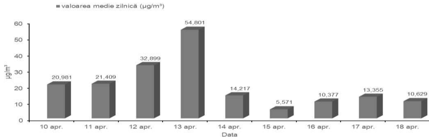
Valorile medii zilnice ale concentrațiilor de particule în suspensie PM2,5 Perioada: 10.04 - 18.04.2021 Depou STB Giurgiului, sector 4
