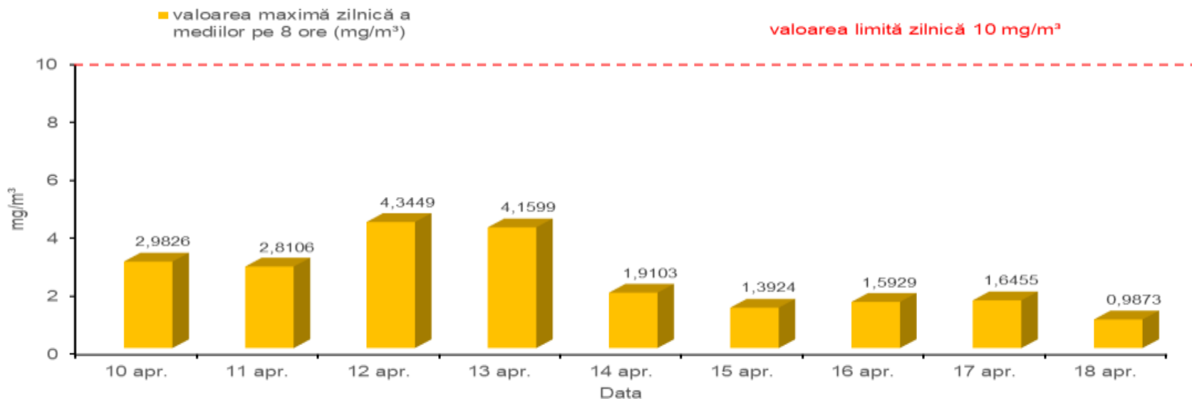
Valorile maxime zilnice a mediilor pe 8 ore ale concentrațiilor de monoxid de carbon (CO) Perioada: 10.04 - 18.04.2021 Depou STB Giurgiului, sector 4
