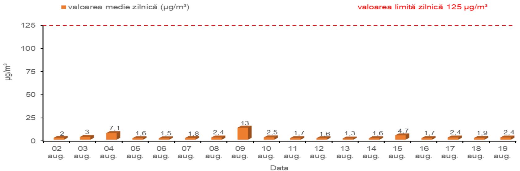
Valorile medii zilnice ale concentrațiilor de dioxid de sulf (SO2) Perioada: 02.08 - 19.08.2018 Lacul Morii, sector 6
