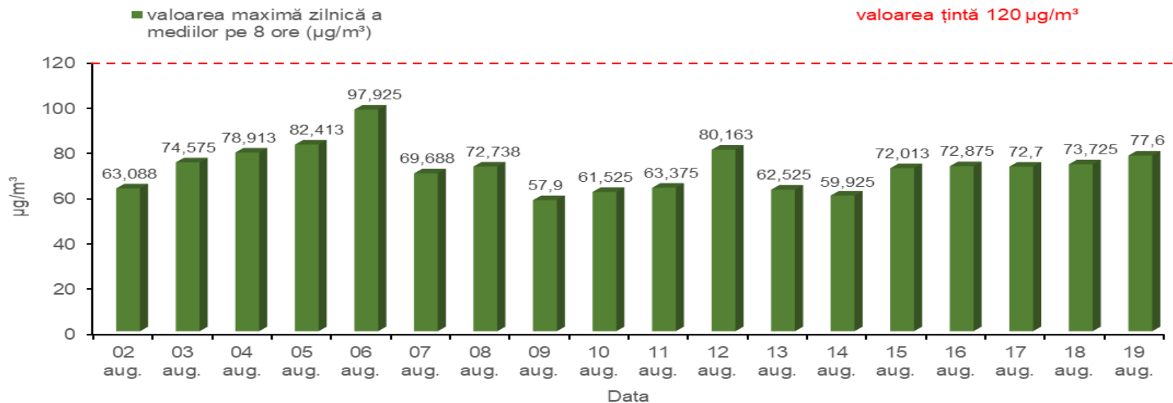
Valorile maxime zilnice a mediilor pe 8 ore ale concentrațiilor de ozon (O3) Perioada: 02.08 - 19.08.2018 Lacul Morii, sector 6
