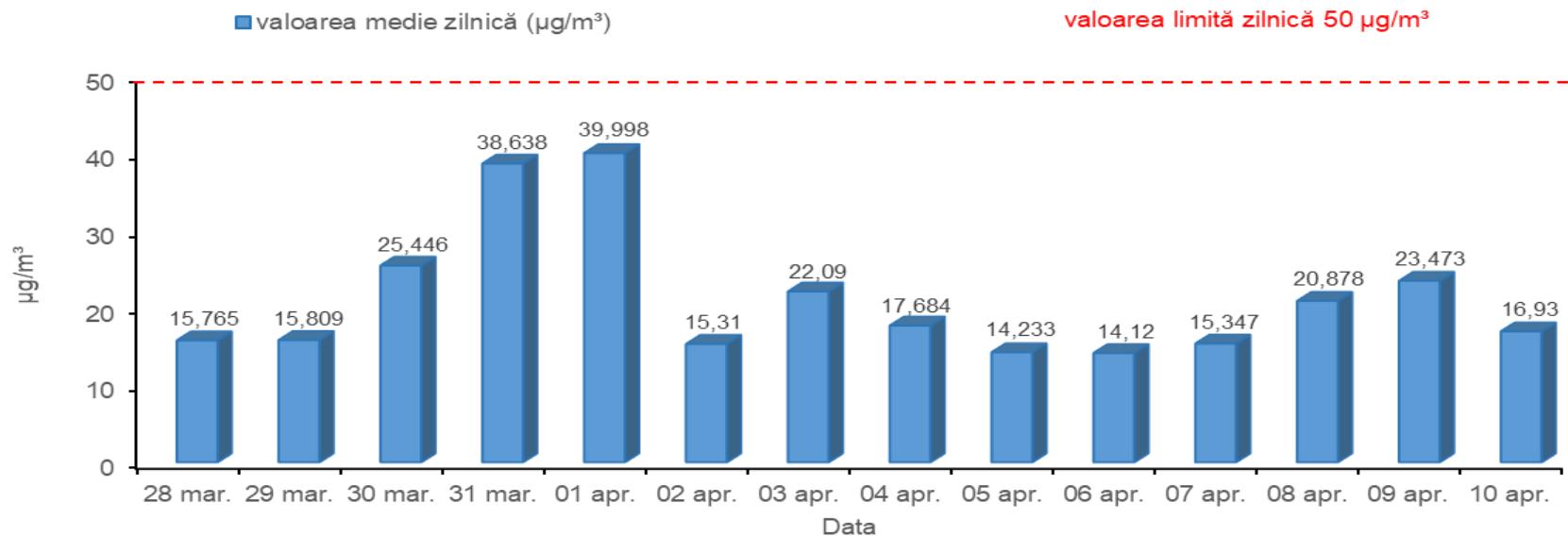
Valorile medii zilnice ale concentrațiilor de particule în suspensie PM10 Perioada: 28.03 - 10.04.2019 Spitalul Clinic Dr. Victor Babeș, sector 3
