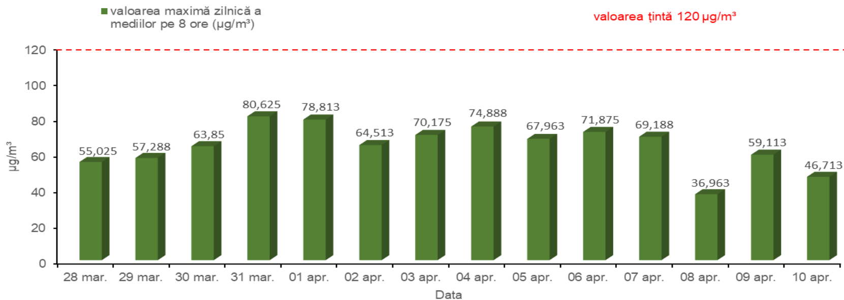
Valorile maxime zilnice a mediilor pe 8 ore ale concentrațiilor de ozon (O3) Perioada: 28.03 - 10.04.2019 Spitalul Clinic Dr. Victor Babeș, sector 3
