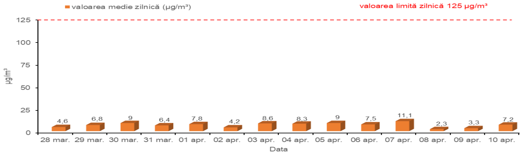
Valorile medii zilnice ale concentrațiilor de dioxid de sulf (SO2) Perioada: 28.03 - 10.04.2019 Spitalul Clinic Dr. Victor Babeș, sector 3
