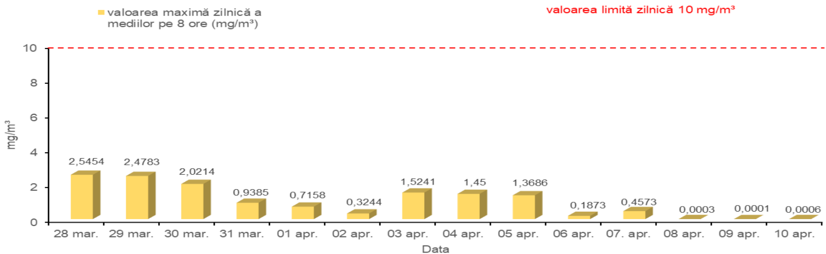
Valorile maxime zilnice a mediilor pe 8 ore ale concentrațiilor de monoxid de carbon (CO) Perioada: 28.03 - 10.04.2019 Spitalul Clinic Dr. Victor Babeș, sector 3
