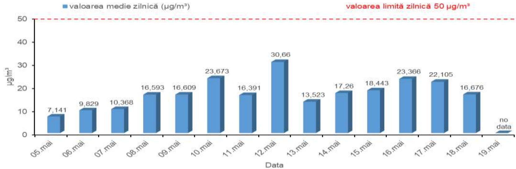
Valorile medii zilnice ale concentrațiilor de particule în suspensie PM10 Perioada: 05.05 - 19.05.2020 Depou STB Nițu Vasile, sector 4
