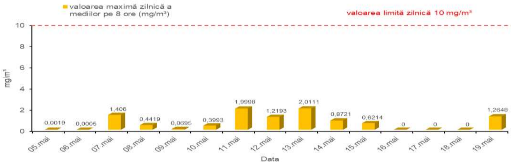
Valorile maxime zilnice a mediilor pe 8 ore ale concentrațiilor de monoxid de carbon (CO) Perioada: 05.05 - 19.05.2020 Depou STB Nițu Vasile, sector 4
