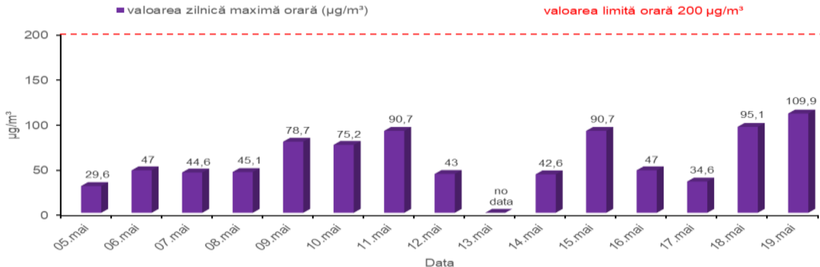
Valorile zilnice maxime orare ale concentrațiilor de dioxid de azot (NO 2 ) Perioada: 05.05 - 19.05.2020 Depou STB Nițu Vasile, sector 4
