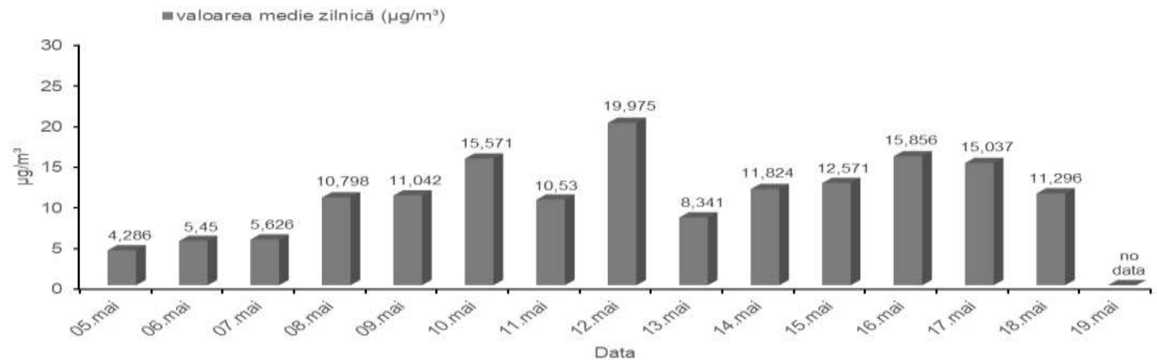
Valorile medii zilnice ale concentrațiilor de particule în suspensie PM2,5 Perioada: 05.05 - 19.05.2020 Depou STB Nițu Vasile, sector 4
