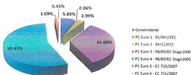
Distributia emisiilor de PM 10 in functie de tehnologie provenite de la autoturisme ce utilizeaza motorina
