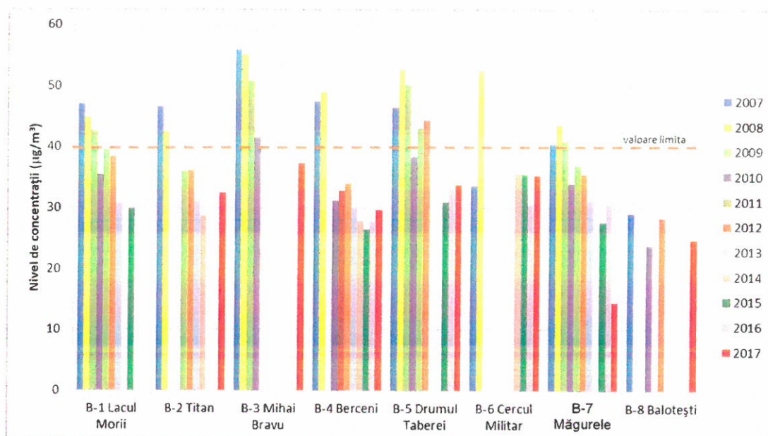
Figura 4.4 Concentrațiile medii anuale pentru PM 10
