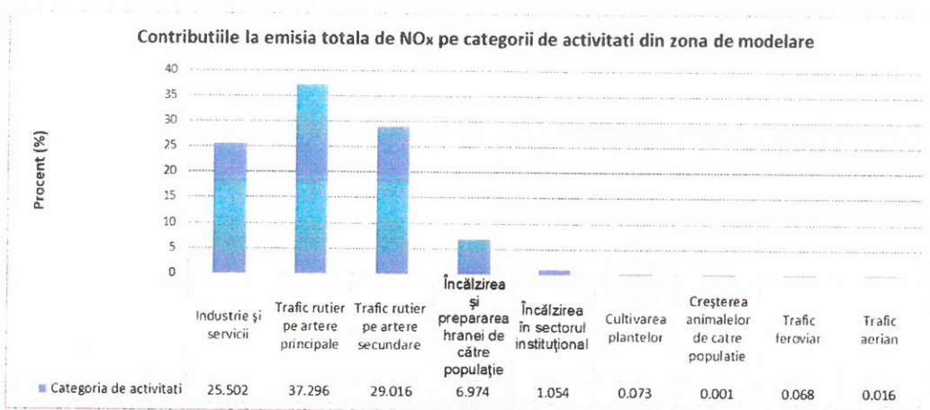
Figura 3.23 Contribuțiile la emisia totală de NO x pe categorii de activități din zona de modelare
