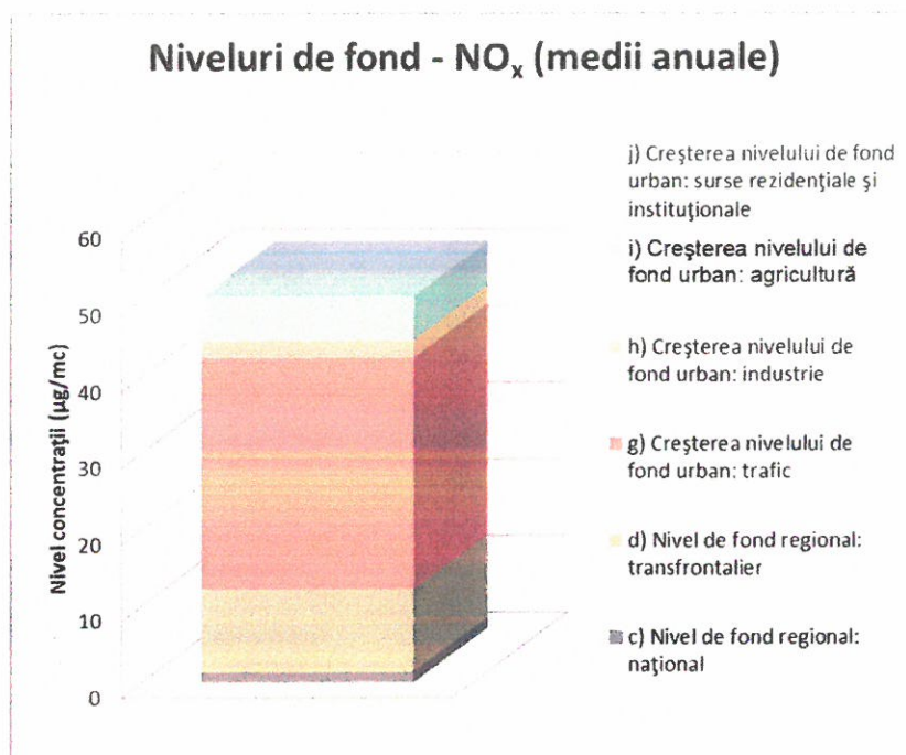
Figura 4.10 Niveluri ale concentrațiilor de fond pentru NO x
