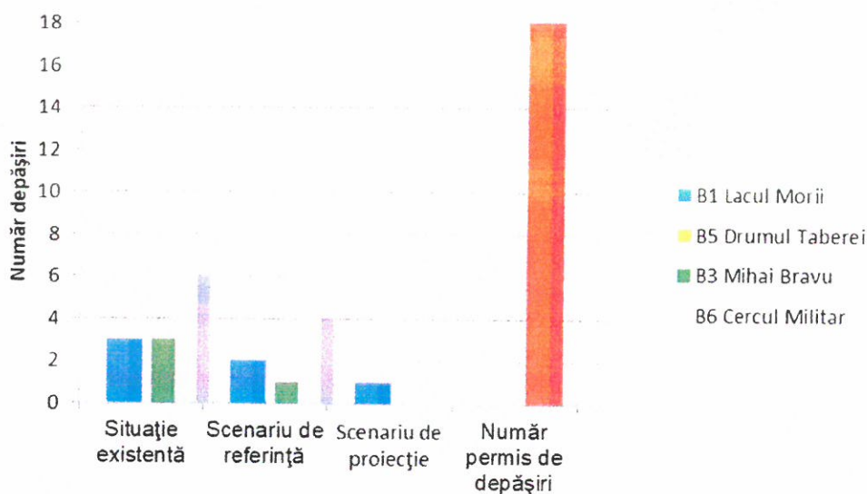
Figura 5.18 Numărul de depășiri anuale ale valorii limită în urma aplicării scenariilor - NO 2
