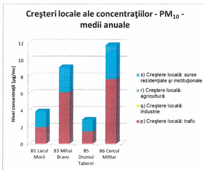
Figura 4.18 Creșteri locale ale concentrațiilor pentru PM 10 - medii anuale
