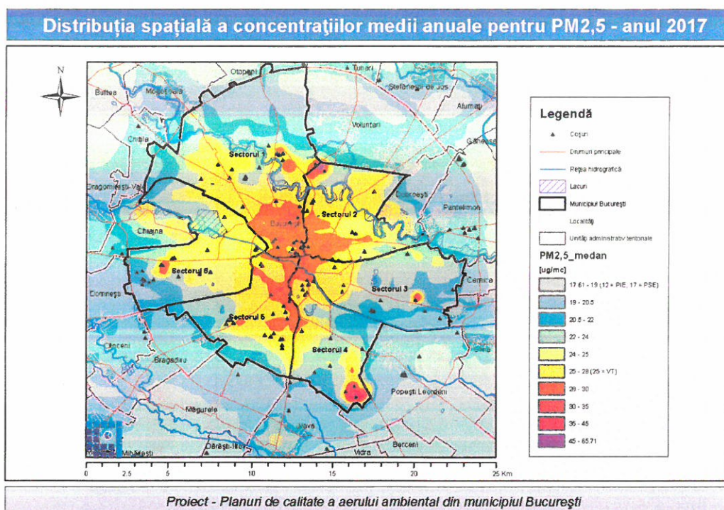
Figura 4.8 Distribuția spațială a concentrațiilor medii anuale pentru PM 2,5
