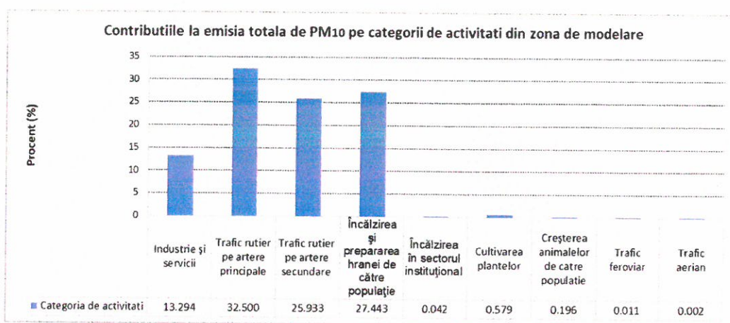
Figura 3.24 Contribuțiile la emisia totală de PM 10 pe categorii de activități din zona de modelare
