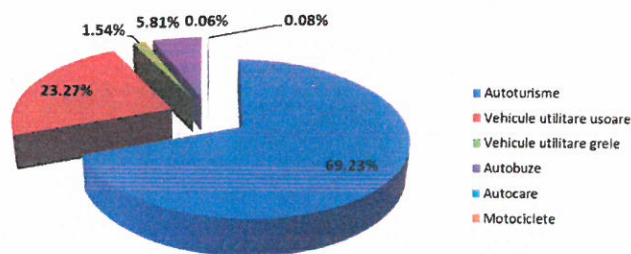
Distributia emisiilor de NO x pe tipuri principale de autovehicule
