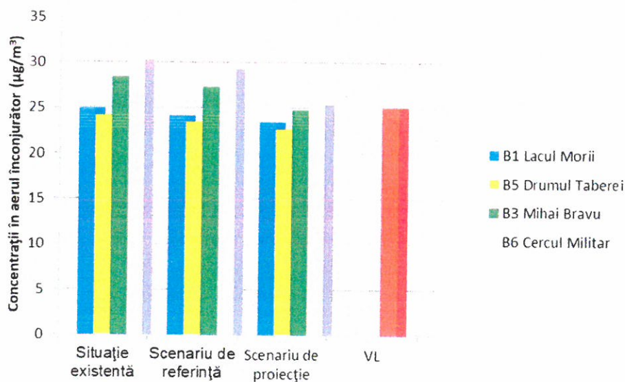
Figura 5.16 Concentrații medii anuale de poluanți în urma aplicării scenariilor - PM 2,5
