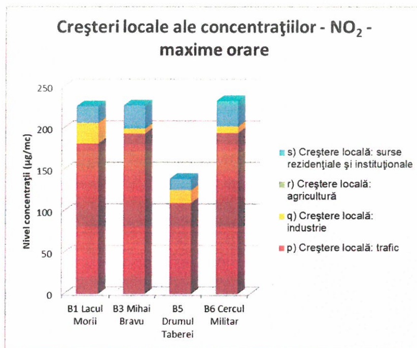
Figura 4.17 Creșteri locale ale concentrațiilor pentru NO 2 - maxime orare
