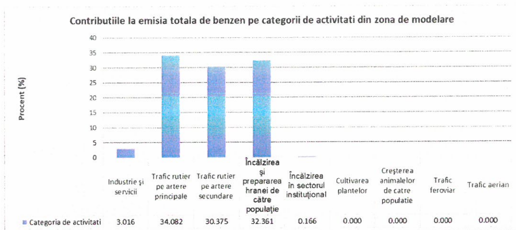
Figura 3.26 Contribuțiile la emisia totală de benzen pe categorii de activități din zona de modelare
