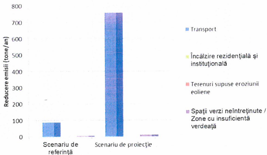
Figura 5.10 Reducerea anuală a emisiilor, pe categorii de surse, în urma aplicării scenariilor - PM 10
