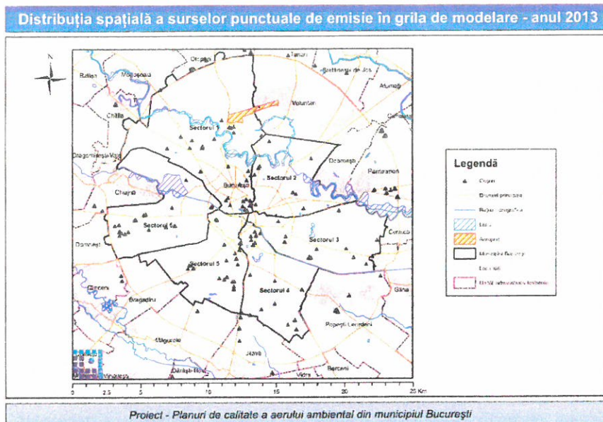
Figura 3.20 Distribuția spațială a surselor punctuale de emisie în grila de modelare - anul 2013
