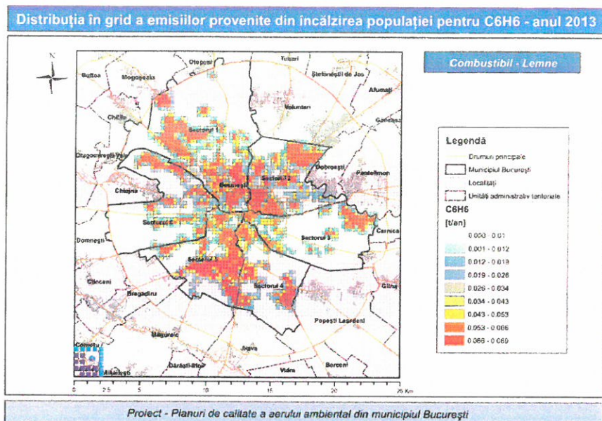
Figura 3.19 Distribuția în grid a emisiilor provenite din încălzirea populației pentru C 6 H 6 (combustibil - lemne) - anul 2013
