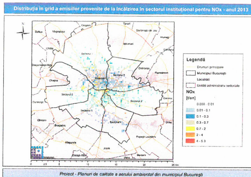
Figura 3.17 Distribuția în grid a emisiilor provenite de la încălzirea în sectorul instituțional pentru NO x - anul 2013
