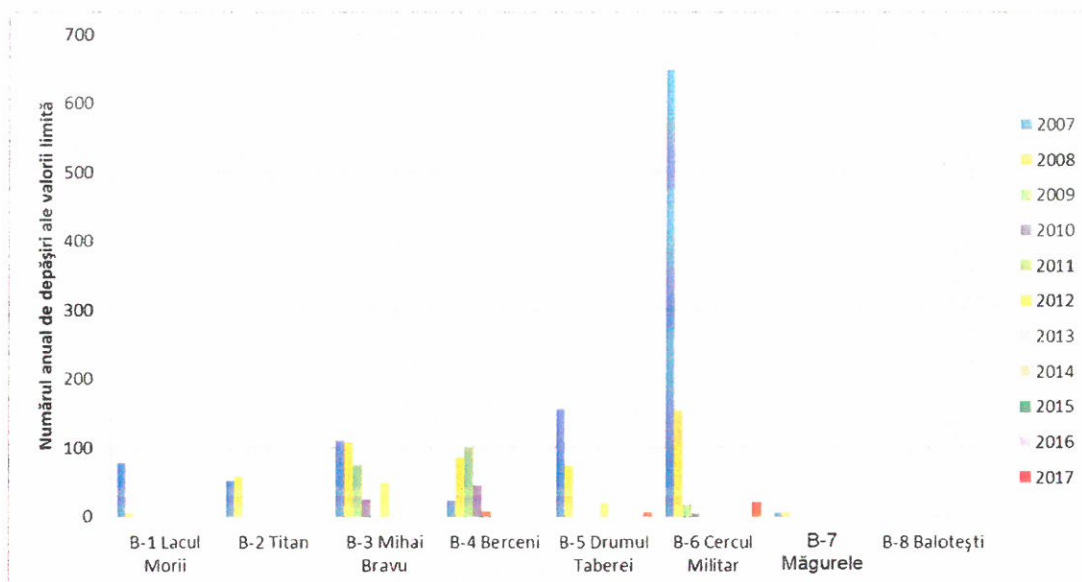
Figura 4.3 Numărul anual de depășiri ale valorii limită pentru dioxidul de azot (NO2)
