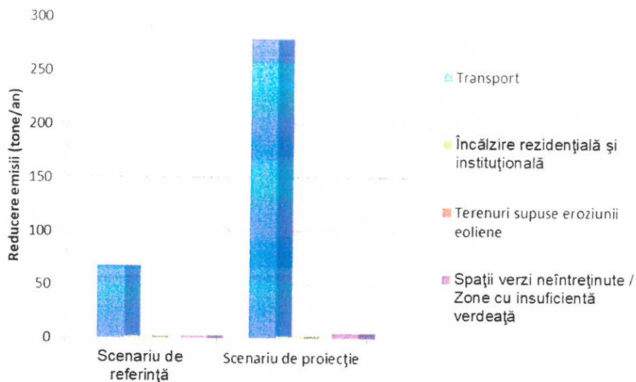
Figura 5.11 Reducerea anuală a emisiilor, pe categorii de surse, în urma aplicării scenariilor - PM_{2,5}
