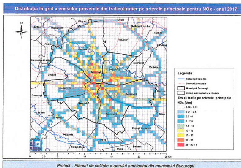
Figura 3.10 Distribuția în grid a emisiilor provenite din traficul rutier pe arterele principale pentru NO x - an de referință
