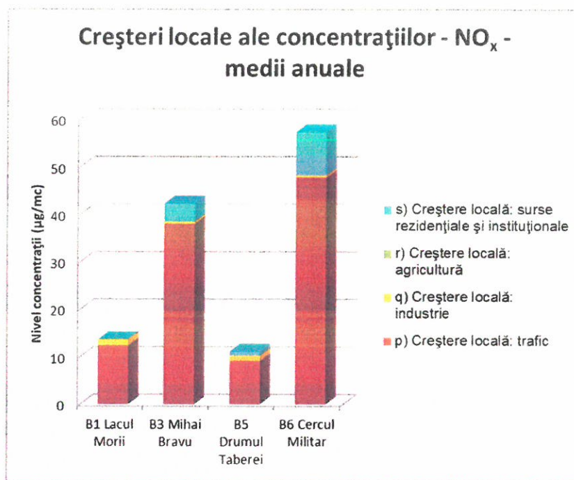
Figura 4.15 Creșteri locale ale concentrațiilor pentru NO x - medii anuale
