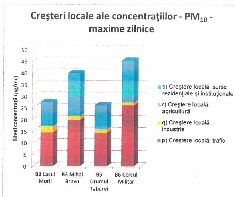
Figura 4.19 Creșteri locale ale concentrațiilor pentru PM 10 - maxime zilnice
