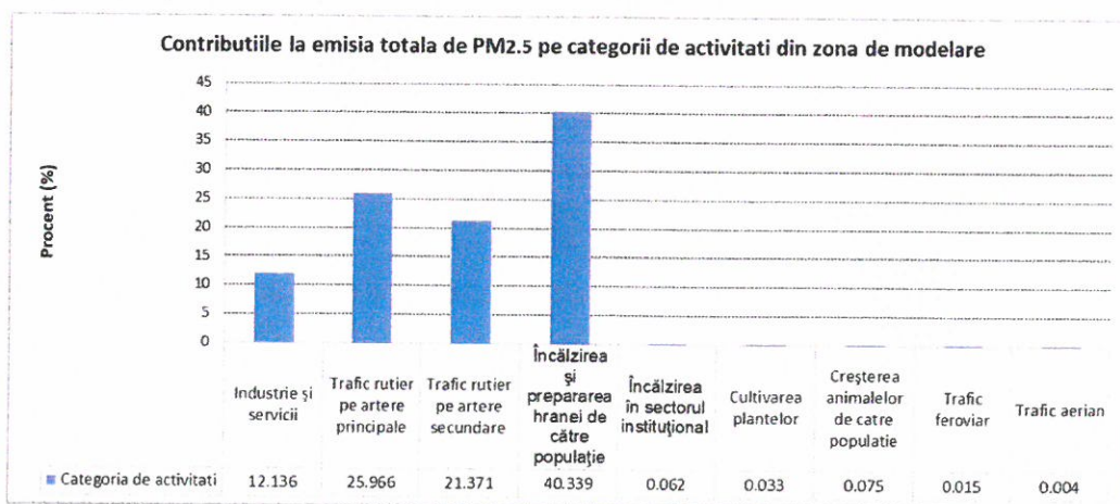
Figura 3.25 Contribuțiile la emisia totală de PM 2.5 pe categorii de activități din zona de modelare
