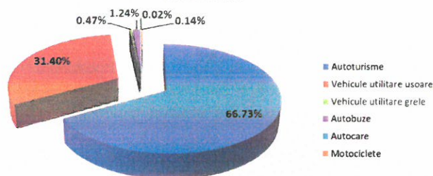
Distribuția emisiilor de PM 10 pe tipuri principale de autovehicule
