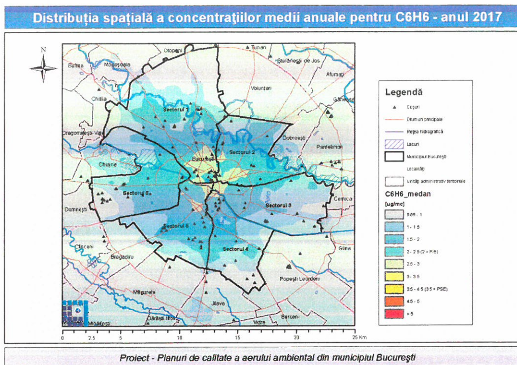
Figura 4.9 Distribuția spațială a concentrațiilor medii anuale pentru C 6 H 6
