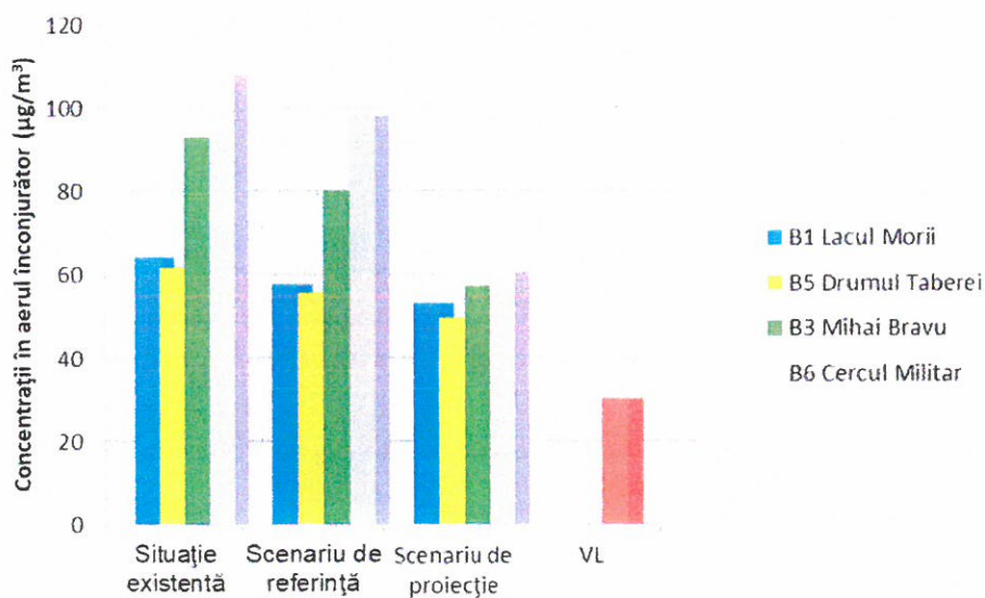
Figura 5.14 Concentrații medii anuale de poluanți în urma aplicării scenariilor - \text{NO}_x
