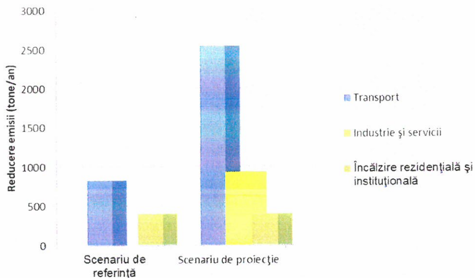
Figura 5.9 Reducerea anuală a emisiilor, pe categorii de surse, în urma aplicării scenariilor - NO x
