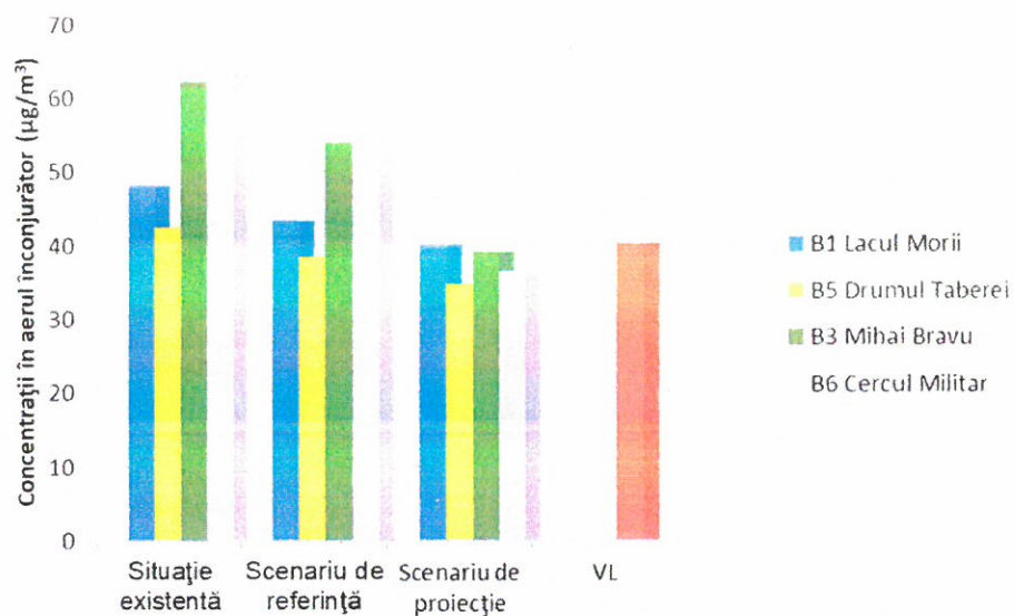
Figura 5.13 Concentrații medii anuale de poluanți în urma aplicării scenariilor - \text{NO}_2
