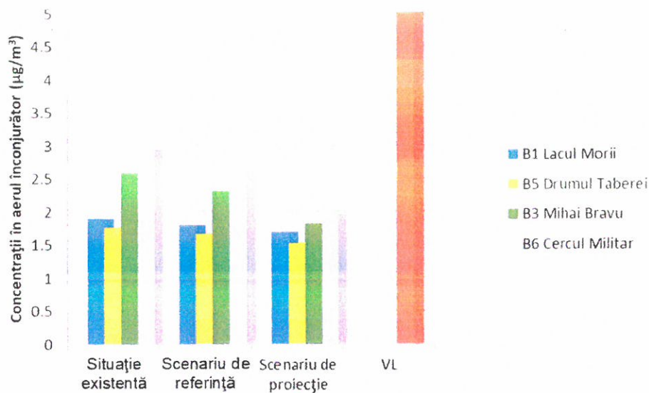
Figura 5.17 Concentrații medii anuale de poluanți în urma aplicării scenariilor - C_6H_6
