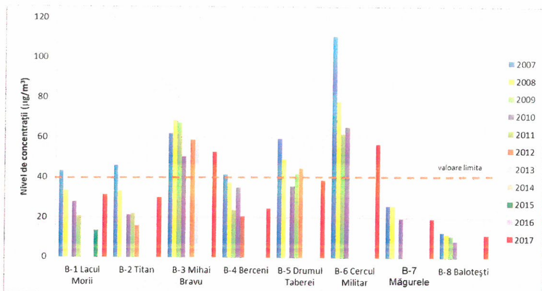
Figura 4.2 Concentrațiile medii anuale pentru dioxidul de azot
