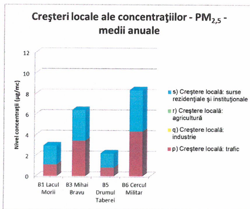
Figura 4.20 Creșteri locale ale concentrațiilor pentru PM 2,5 - medii anuale
