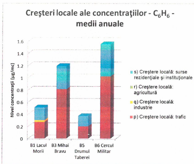
Figura 4.21 Creșteri locale ale concentrațiilor pentru C_6H_6 - medii anuale
