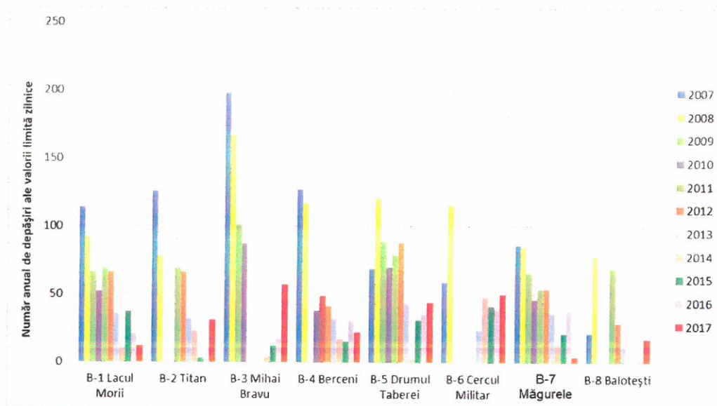
Figura 4.5 Numărul anual de depășiri ale valorii limită zilnice pentru PM_{10}
