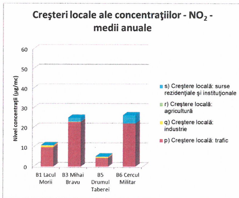
Figura 4.16 Creșteri locale ale concentrațiilor pentru NO 2 - medii anuale
