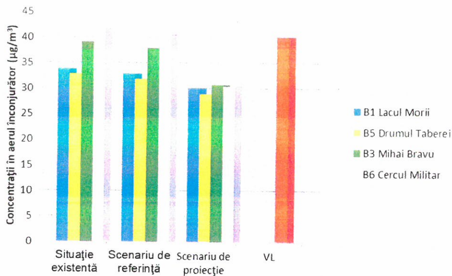
Figura 5.15 Concentrații medii anuale de poluanți în urma aplicării scenariilor - PM 10
