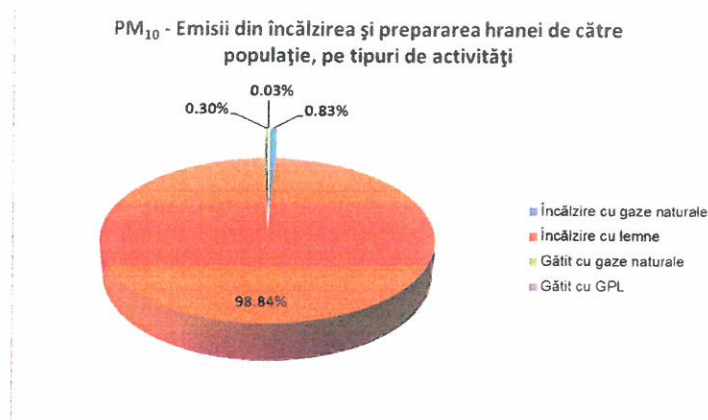
Figura 3.14 PM 10 - emisii din încălzirea și prepararea hranei de către populație în municipiul București
