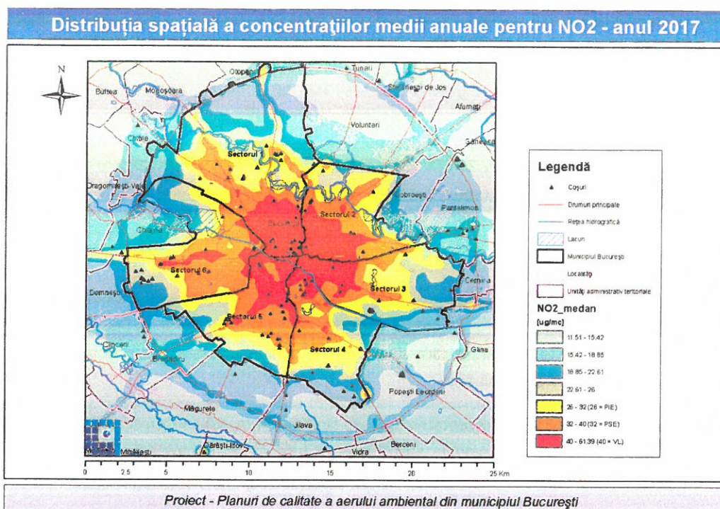
Figura 4.6 Distribuția spațială a concentrațiilor medii anuale pentru NO 2
