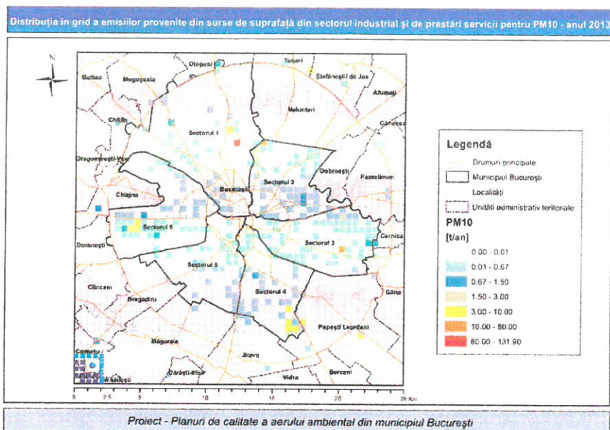
Figura 3.22 Distribuția în grid a emisiilor provenite din surse de suprafață din sectorul industrial și de prestări servicii pentru PM 10 - anul 2013
