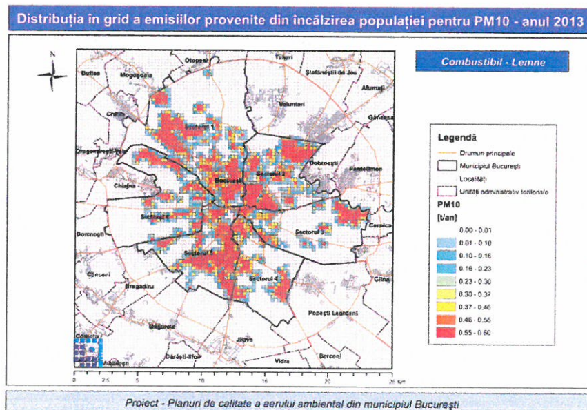
Figura 3.18 Distribuția în grid a emisiilor provenite din încălzirea populației pentru PM 10 (combustibil - lemne) - anul 2013
