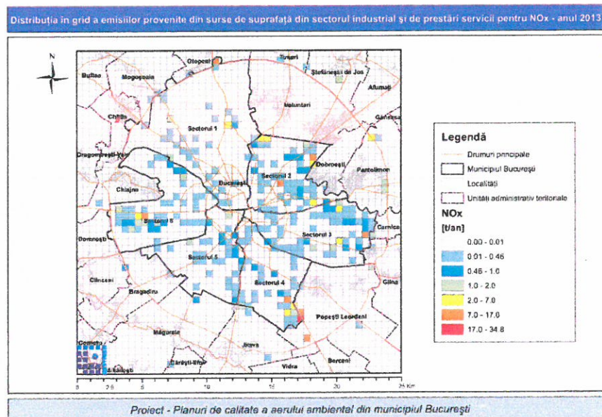
Figura 3.21 Distribuția în grid a emisiilor provenite din surse de suprafață din sectorul industrial și de prestări servicii pentru NO x - anul 2013
