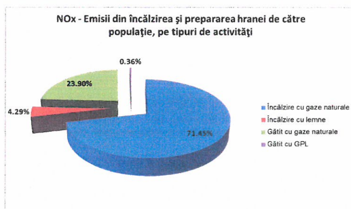
Figura 3.13 NO x - emisii din încălzirea și prepararea hranei de către populație în municipiul București
