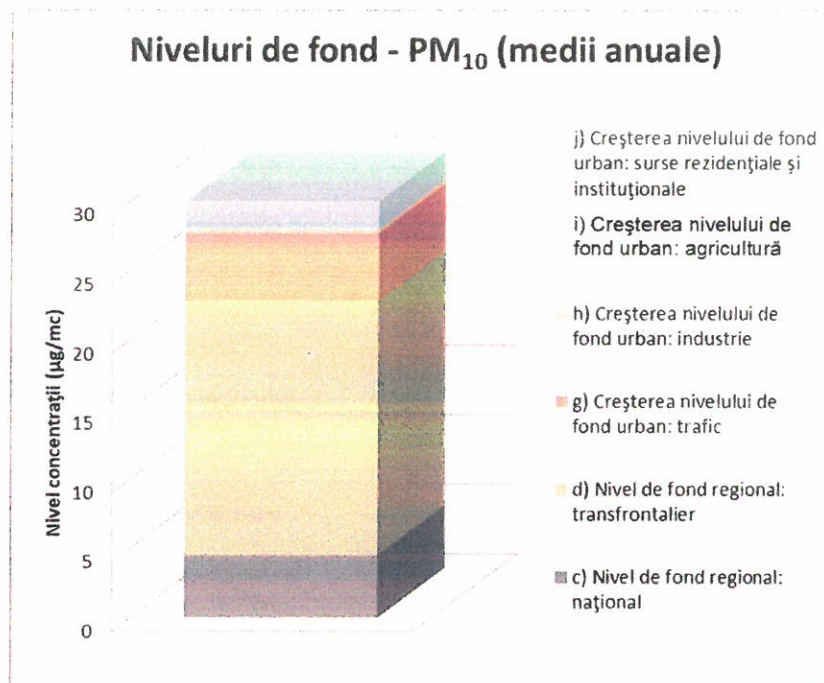
Figura 4.12 Niveluri ale concentrațiilor de fond pentru PM 10
