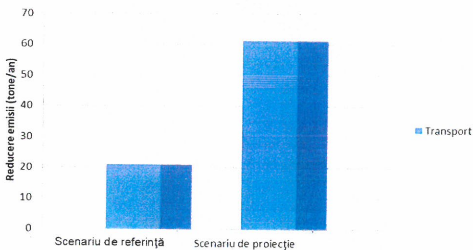
Figura 5.12 Reducerea anuală a emisiilor, pe categorii de surse, în urma aplicării scenariilor - C_6H_6
