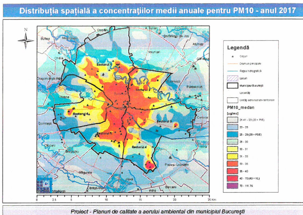
Figura 4.7 Distribuția spațială a concentrațiilor medii anuale pentru PM 10
