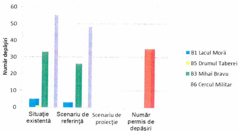
Figura 5.19 Numărul de depășiri anuale ale valorii limită în urma aplicării scenariilor - PM 10
