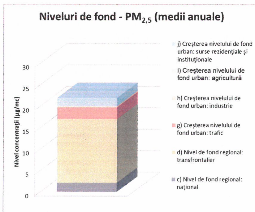
Figura 4.13 Niveluri ale concentrațiilor de fond pentru PM 2,5
