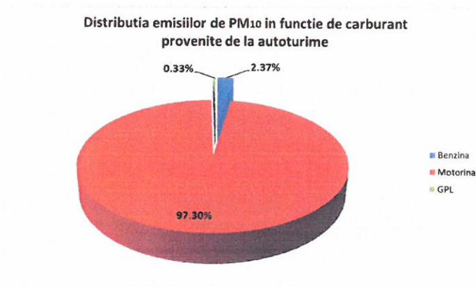
Figura 3.6 Distribuția emisiilor de PM 10 în funcție de carburant provenite de la autoturisme
