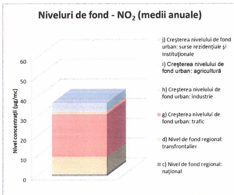
Figura 4.11 Niveluri ale concentrațiilor de fond pentru NO 2
