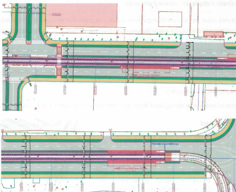
Figură 103 - Propunere de amenajare a Bd-ului. Dimitrie Pompeiu (secțiuni relevante)
