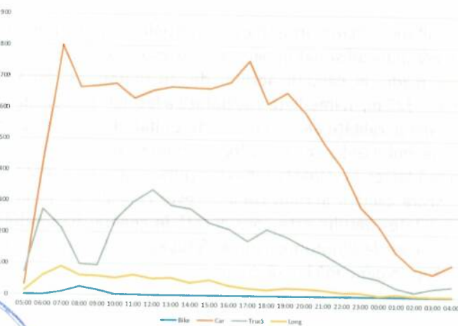
Figură 36 - Variația orară a fluxurilor de trafic, anul 2024 – valori orare, postul 17 (secțiune)
