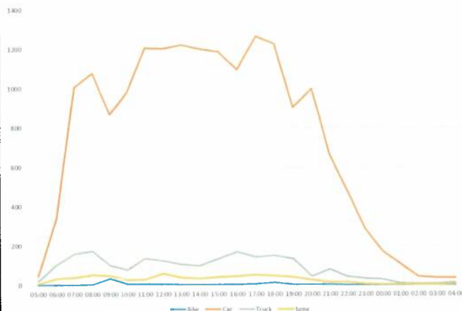
Figură 26 - Variația orară a fluxurilor de trafic, anul 2024 – valori orare, postul 7 (secțiune)
