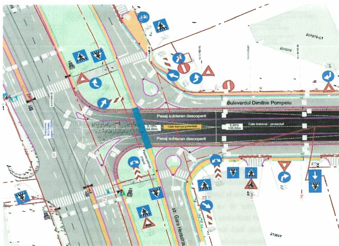
Propunere amenajare intersecție dintre Bld Barbu Vacarescu și Bld Dimitrie Pompeiu
