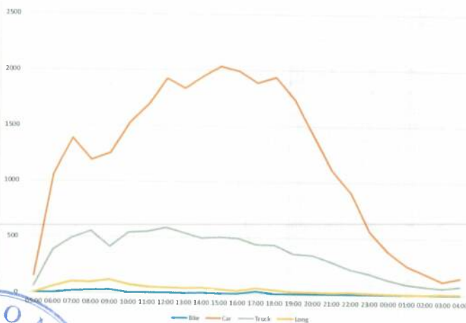
Figură 30 - Variația orară a fluxurilor de trafic, anul 2024 – valori orare, postul 11 (secțiune)
