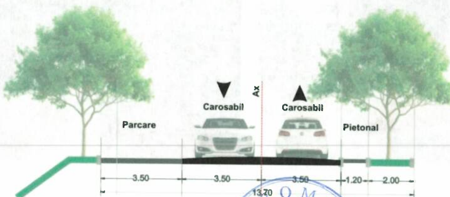
Figură 16 - Secțiune transversală prin strada Gara Herăstrău (în partea sudică a b-dului Dimitrie Pompeiu)
