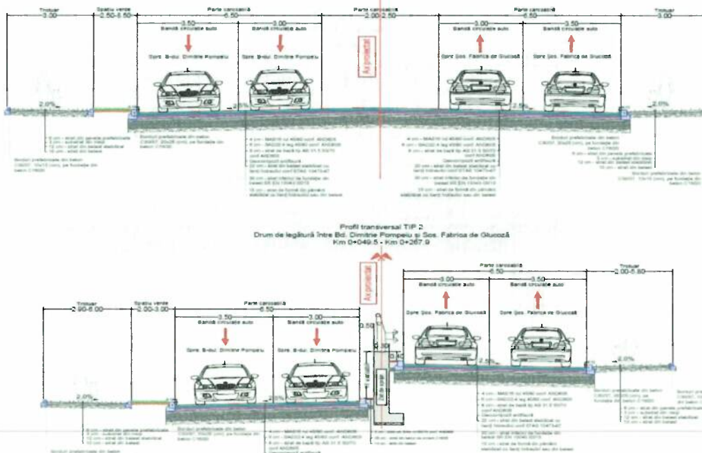
Profile transversale tip propuse pe drum de legatura bld D. Pompeiu si Fabrica de Glucoza
