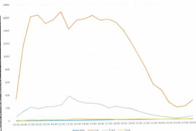
Figură 20 - Variația orară a fluxurilor de trafic, anul 2024 – valori orare, postul 1 (secțiune)
