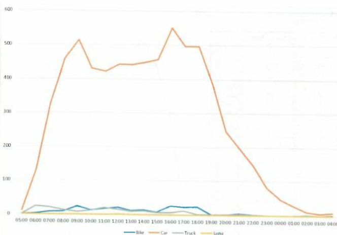
Figură 29 - Variația orară a fluxurilor de trafic, anul 2024 – valori orare, postul 10 (secțiune)
