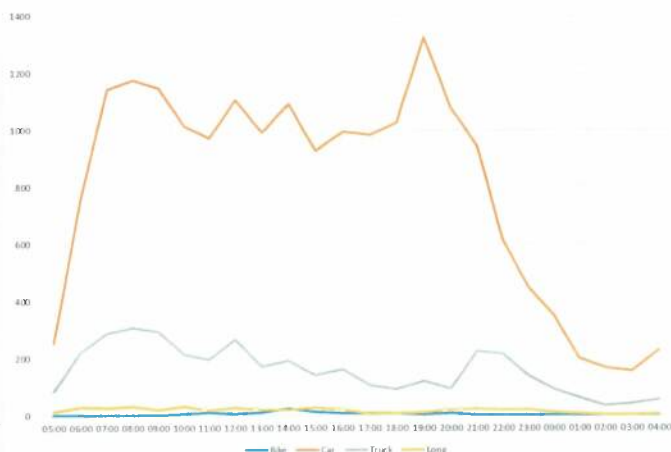
Figură 25 - Variația orară a fluxurilor de trafic, anul 2024 – valori orare, postul 6 (secțiune)
