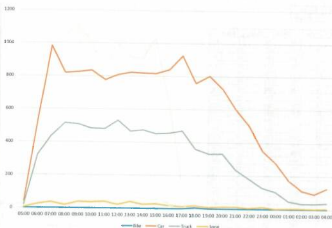
Figură 28 - Variația orară a fluxurilor de trafic, anul 2024 – valori orare, postul 9 (secțiune)
