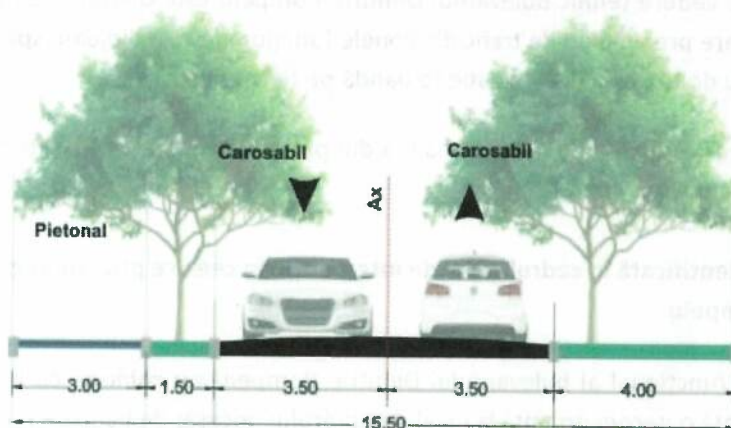
Figură 9 - Secțiune transversală prin b-dul Dimitrie Pompeiu (spre str. Petricani)
