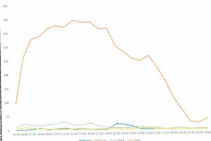
Figură 21 - Variația orară a fluxurilor de trafic, anul 2024 – valori orare, postul 2 (secțiune)
