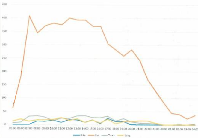
Figură 23 - Variația orară a fluxurilor de trafic, anul 2024 – valori orare, postul 4 (secțiune)
