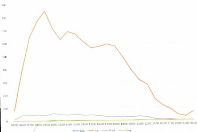
Figură 33 - Variația orară a fluxurilor de trafic, anul 2024 – valori orare, postul 14 (secțiune)
