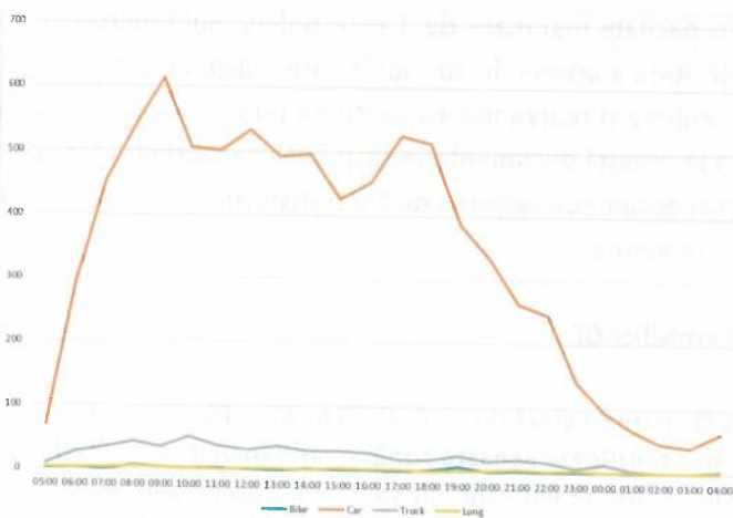
Figură 35 - Variația orară a fluxurilor de trafic, anul 2024 – valori orare, postul 16 (secțiune)
