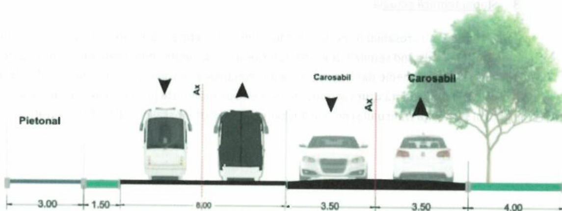
Figură 10 - Secțiune transversală prin b-dul Dimitrie Pompeiu (spre str. Gara Herastrau), cu liniile de tramvai
