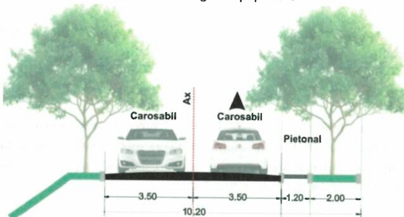
Figură 15 - Secțiune transversală prin strada Gara Herăstrău (tronson între Șoseaua Pipera și Bulevardul Dimitriei Pompeiu)
