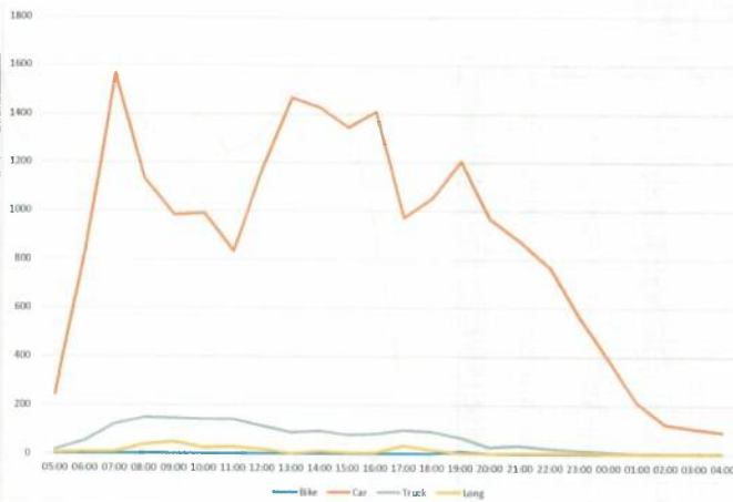
Figură 22 - Variația orară a fluxurilor de trafic, anul 2024 – valori orare, postul 3 (secțiune)
