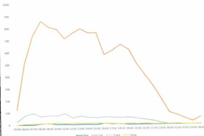
Figură 32 - Variația orară a fluxurilor de trafic, anul 2024 – valori orare, postul 13 (secțiune)
