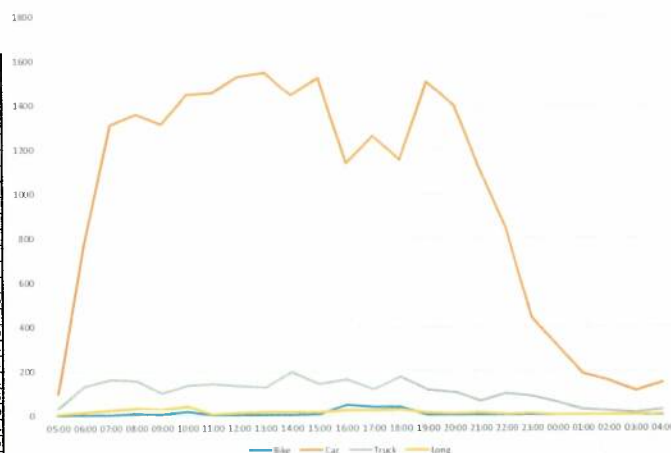
Figură 27 - Variația orară a fluxurilor de trafic, anul 2024 – valori orare, postul 8 (secțiune)
