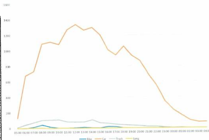
Figură 37 - Variația orară a fluxurilor de trafic, anul 2024 – valori orare, postul 18 (secțiune)
