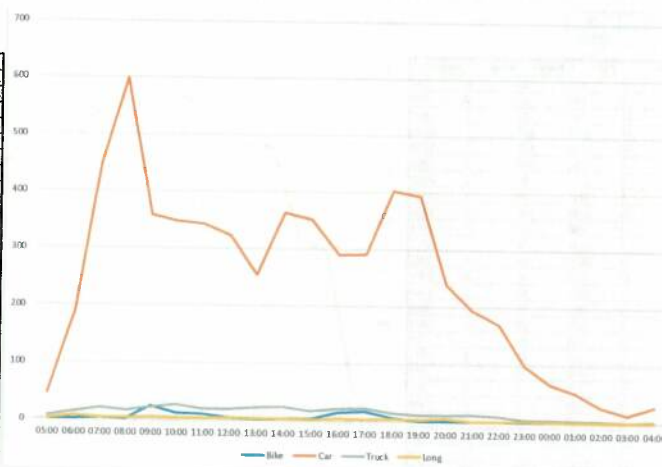
Figură 34 - Variația orară a fluxurilor de trafic, anul 2024 – valori orare, postul 15 (secțiune)
