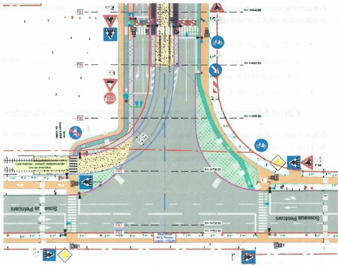
Propunere amenajare intersecție dintre Bld Dimitrie Pompeiu și Soseaua Petricani
