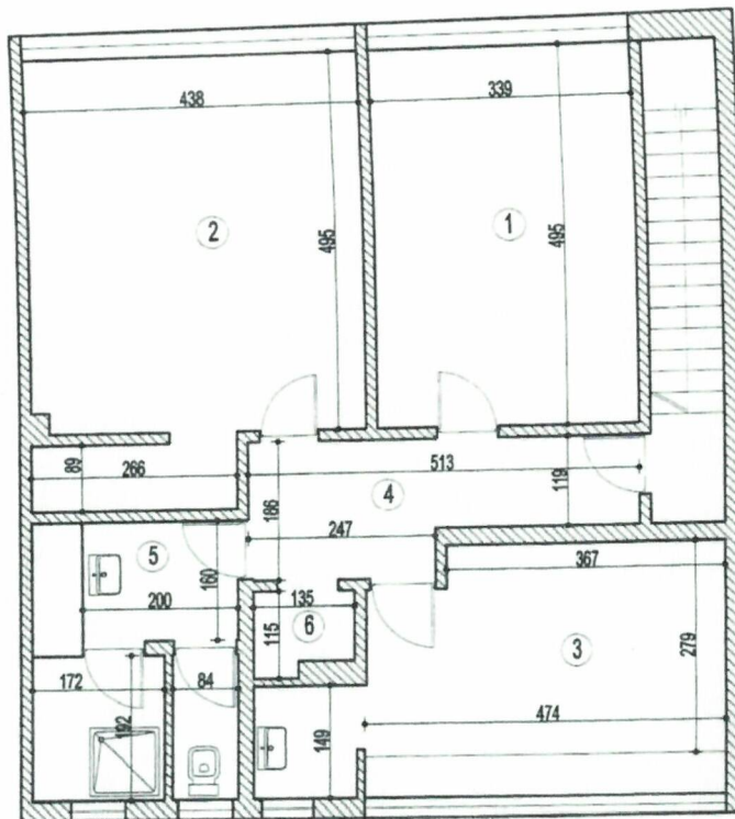
PLAN ETAJ 1 _ Spatiu cu Alta Destinatie
