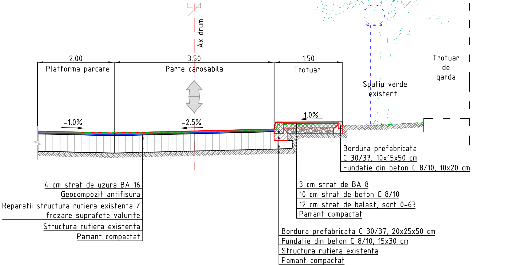
PROFIL TRANSVERSAL TIP 06 Scara 1 : 50
