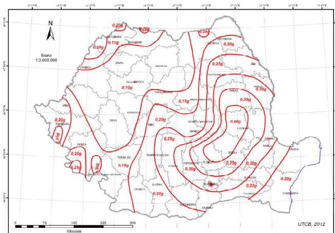
Zonarea teritoriului României în termeni de valori de vârf ale accelerației terenului pentru proiectare a_g pentru cutremure având intervalul mediu de recurența IMR = 225 ani și 20% posibilitate de depășire în 50 de ani.
